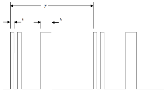
Figura X – Emisiones pulsadas con dos diferentes duraciones en los pulsos (por ejemplo si, t_1= 1 ms, t_2= 5 ms, a_1=2 , a_2=1 , T= 25 ms, entonces \delta(\text{dB}) = -11,06 \text{ dB} )
