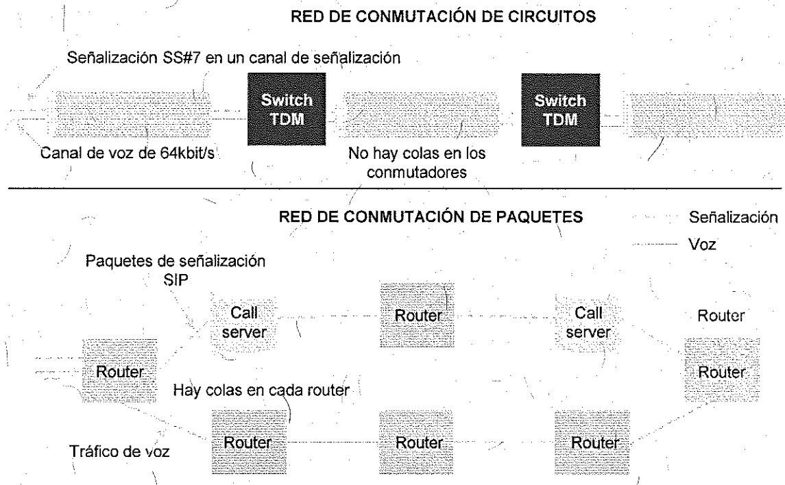
Figura 2: Comparación entre redes de conmutación de circuitos y de conmutación de paquetes (Fuente: Analysys Mason, 2016)
