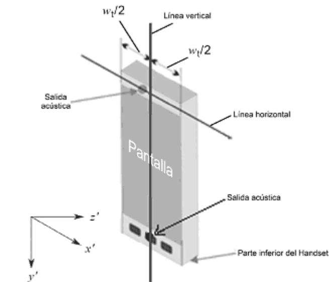
Figura N.2 - Ejemplo de sistema de coordenadas en el Equipo Bajo Prueba
