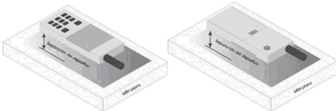
Figura 18. Posiciones de prueba para DUC.
