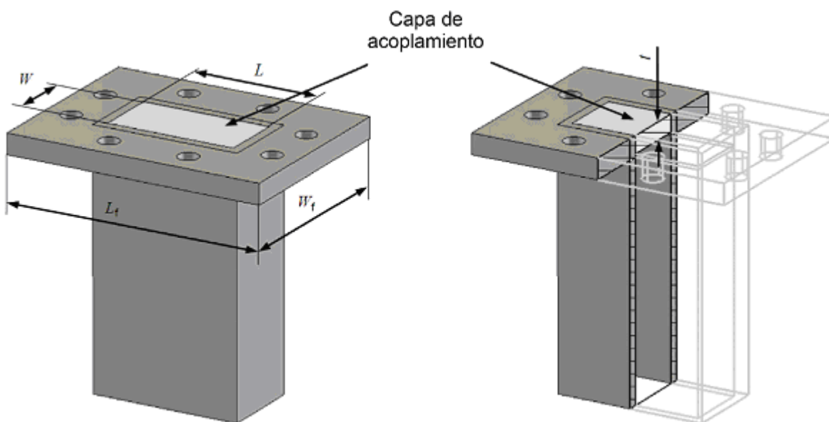
Figura Q.2.- Guía de onda estándar como fuente (dimensiones están de acuerdo a la tabla Q.2)
