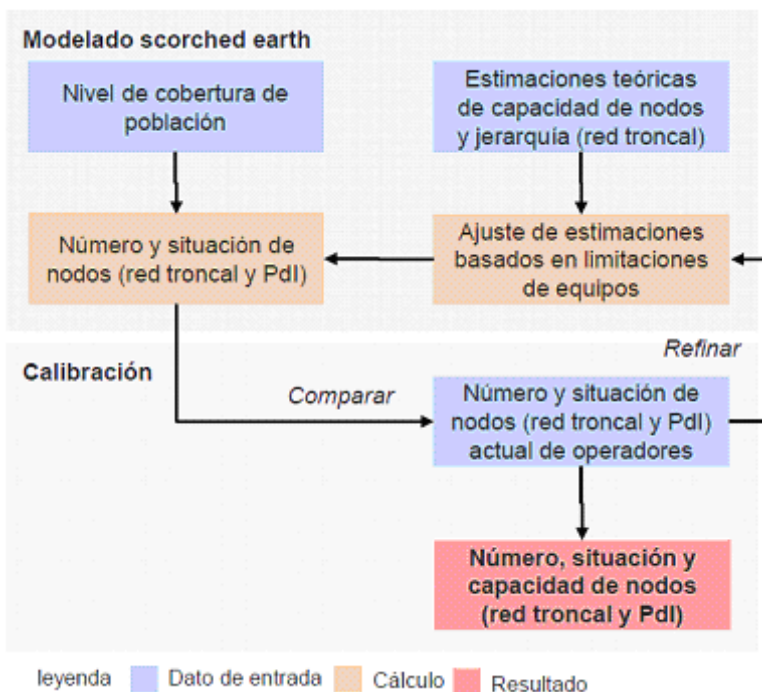
Figura 4: Esquema de modelado scorched-earth calibrado para el operador fijo [Fuente: Analysys Mason, 2012] A continuación se muestra un esquema con la metodología utilizada para la calibración del Modelo Móvil.
