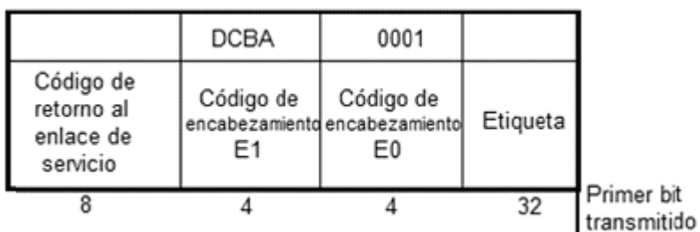
FIGURA 36.- Mensaje de retorno al enlace de servicio.
