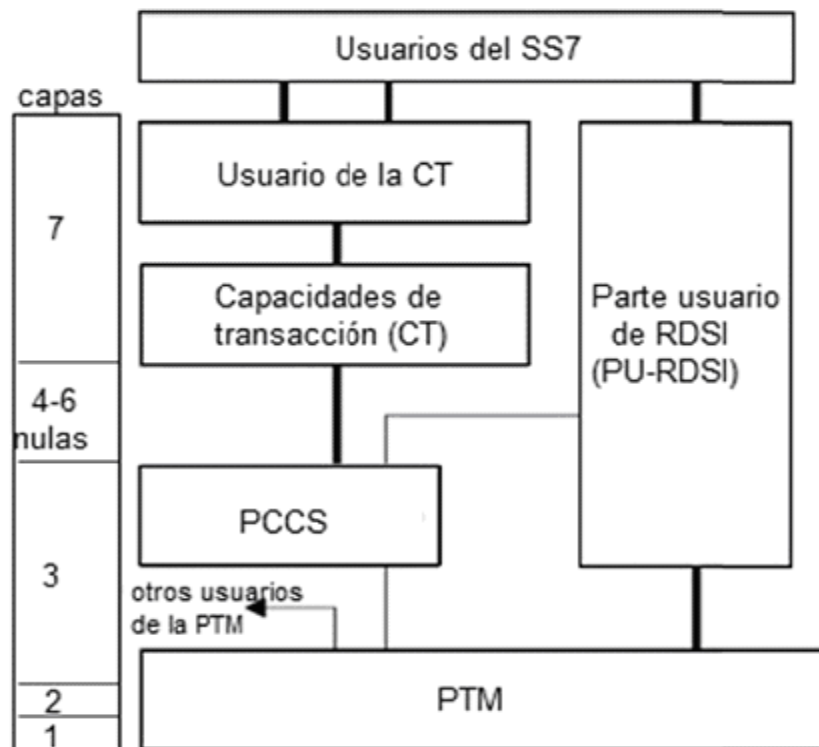
FIGURA 2.- Arquitectura del sistema de señalización N.º 7.
