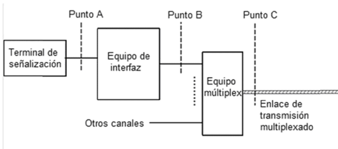
b) Ejemplo 2.- Enlace de datos de señalización (digital o analógico) mediante equipo de interfaz
