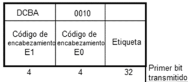
FIGURA 37.- Mensaje de paso de emergencia a enlace de reserva.
