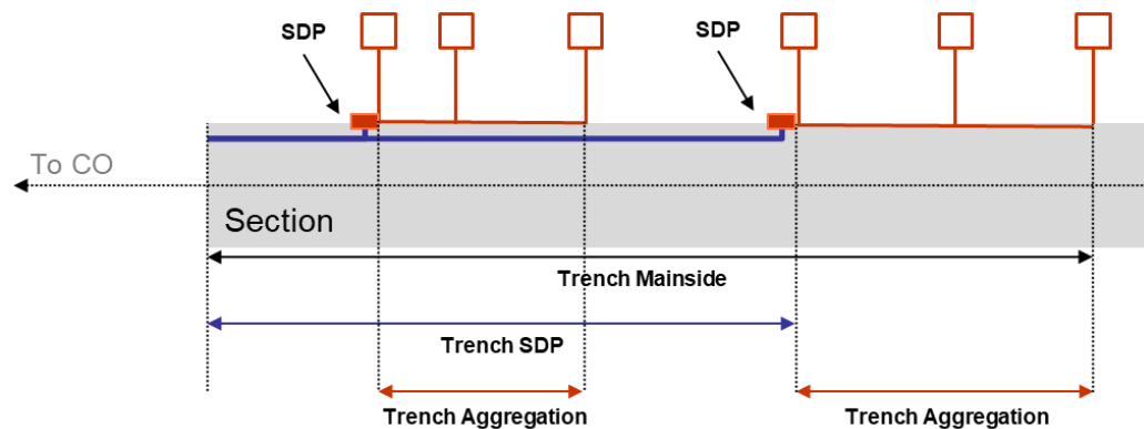
Figura 42 - asignación de longitud de zanjas
