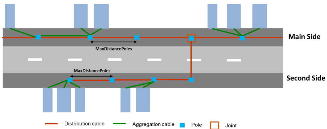
Figura 39 Ubicación de los postes
