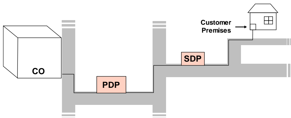
Figura 21 - Arquitectura de red de FTTH (solo para fines ilustrativos)
