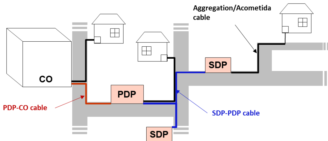
Figura 31 Tipos de cables que pasan por una sección
