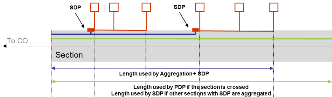
Figura 41 Longitud de la zanja utilizada por los diferentes niveles de la red
