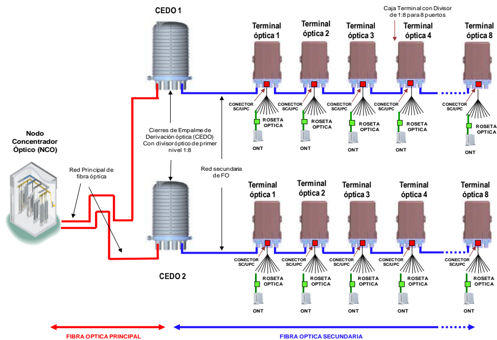
Figura 22 - Niveles de división de la red de fibra
