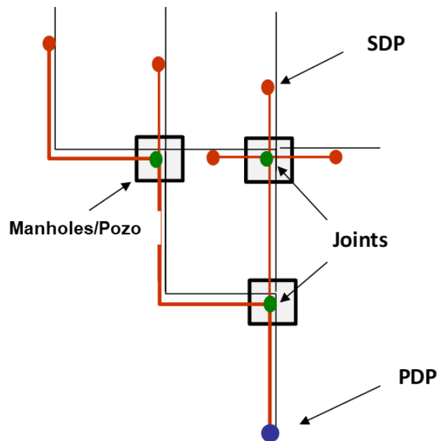
Figura 38 Cierres y pozos
