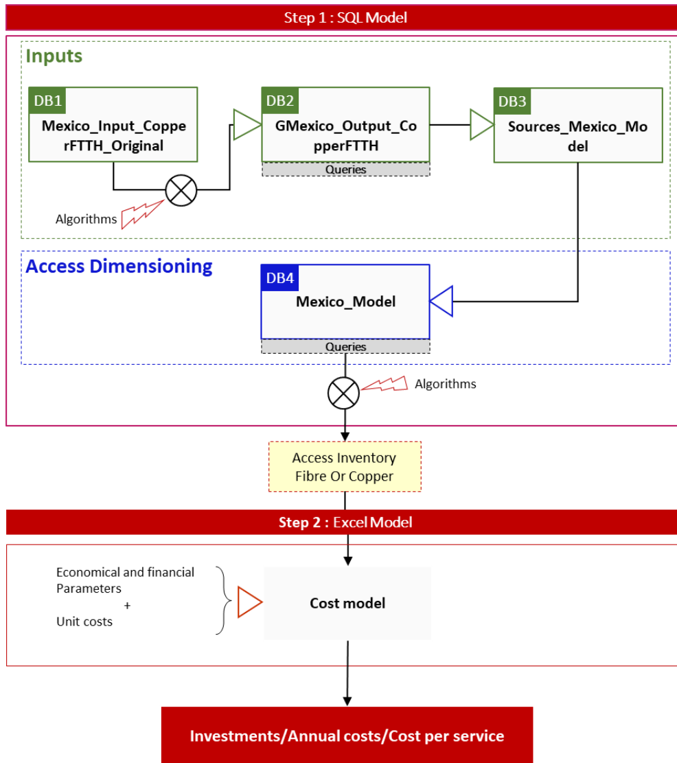
Figura 13 – Arquitectura general del módulo SQL
