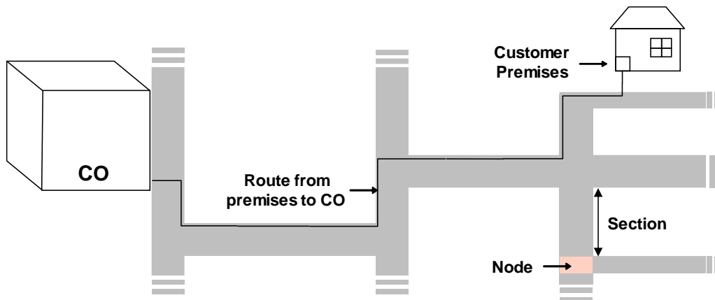
Figura 16 - Secciones de camino
