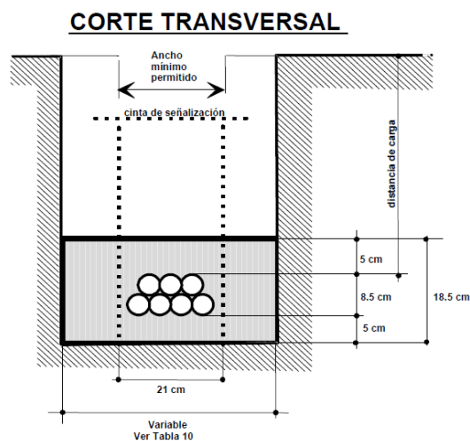
Figura 35 Ejemplo de "Canalizaciones" usadas como zanjas + conductos tipo 7H4
