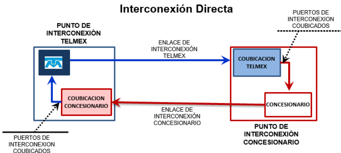
Diagrama de Interconexión con protocolo SIP
