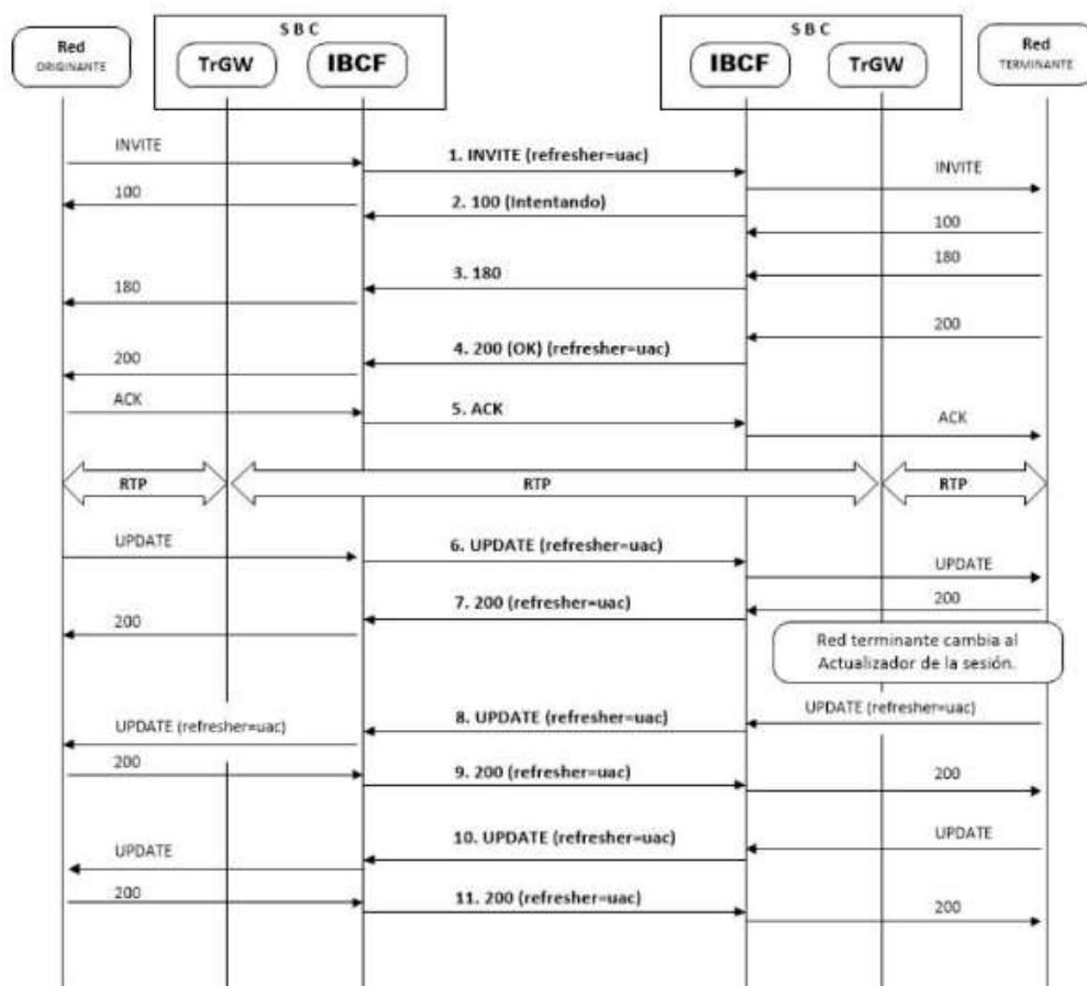
Diagrama 3. Actualización de sesión.
