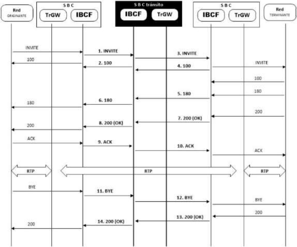
Diagrama 5. Establecimiento de una llamada de tránsito.
