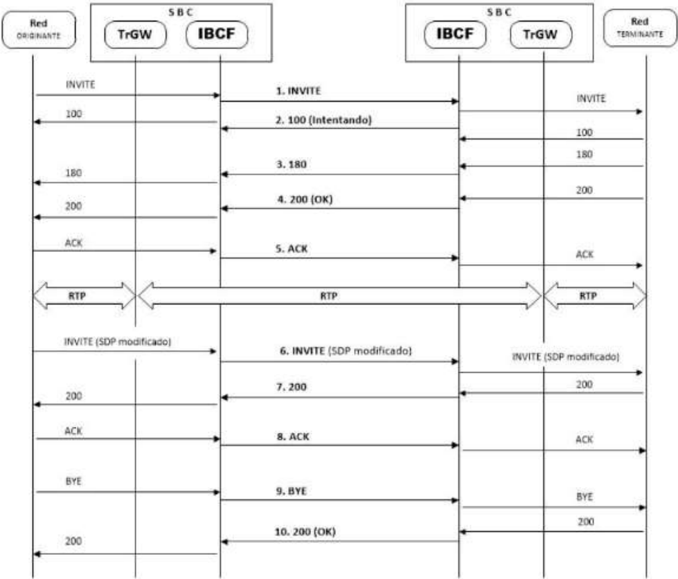
Diagrama 4. Actualización del medio.
