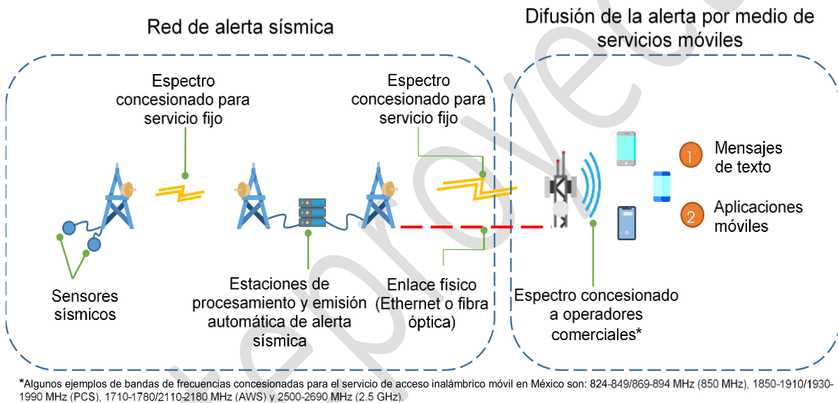
Figura 2. Alternativa de difusión de alerta a dispositivos celulares
