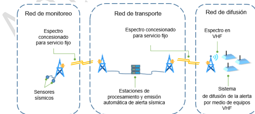
Figura 8. Esquema de distribución del sistema de alerta sísmica, elaborado por el Instituto.
