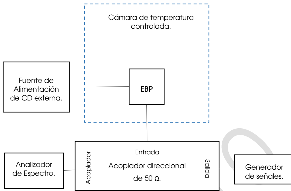
Figura 3. Ejemplo de Conexión típica de la instrumentación y EBP para la prueba de Tolerancia en frecuencia.
