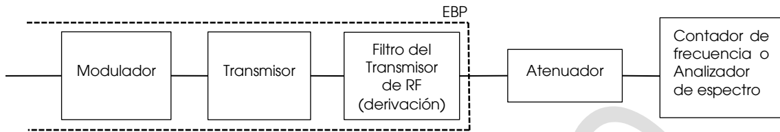
Figura 6. Configuración de prueba conducida para la exactitud en frecuencia.
