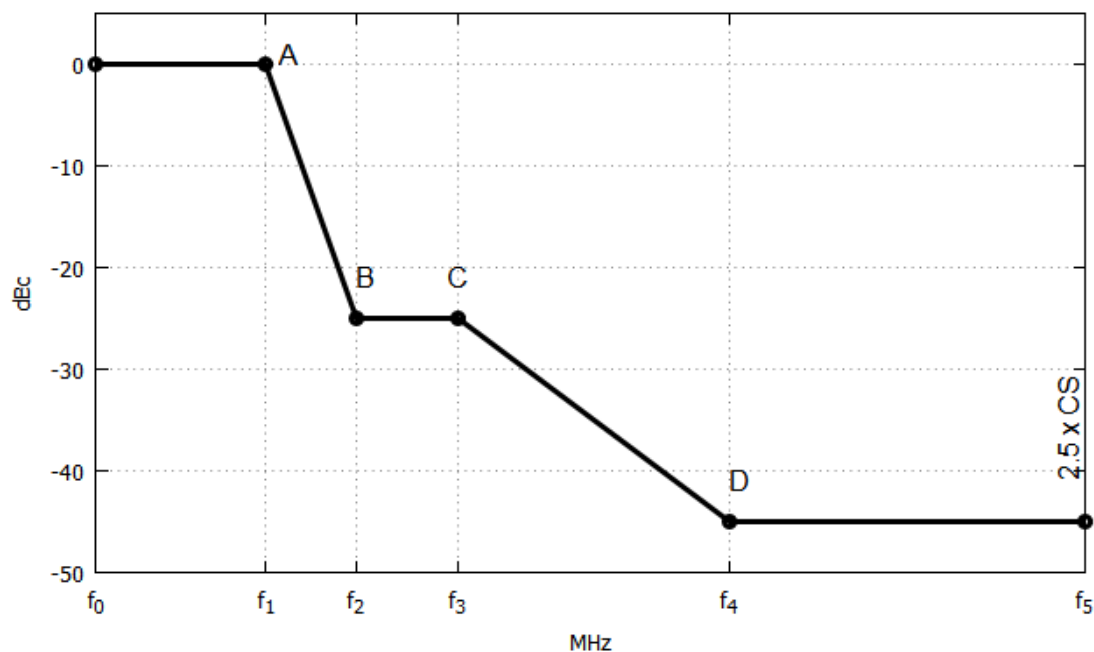
Figura 4. Contorno de las Emisiones fuera de banda.
