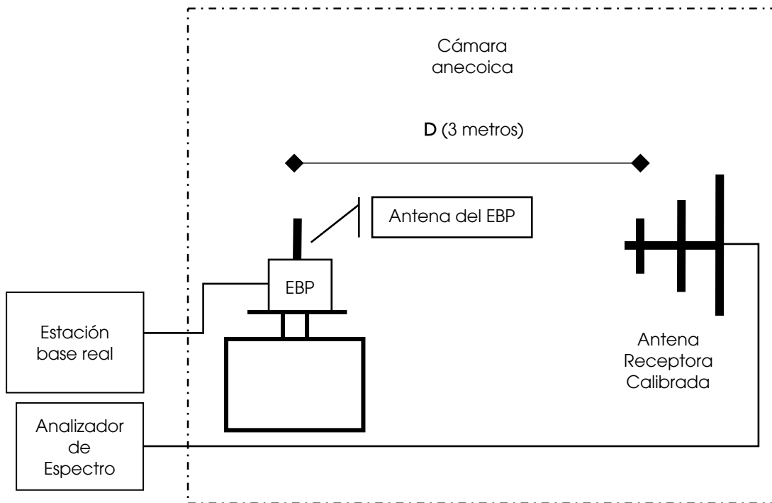
Figura 3. Configuración para medición de emisiones radiadas.
