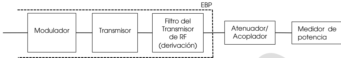
Figura 5. Configuración de prueba conducida para la potencia media de RF.
