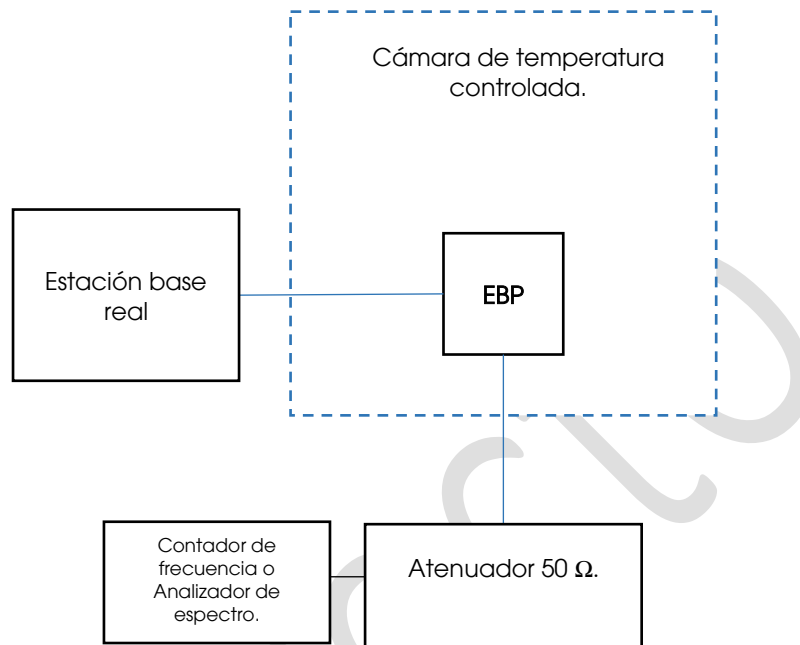
Figura 7. Conexión típica de la instrumentación y EBP para la prueba de Tolerancia en frecuencia.
