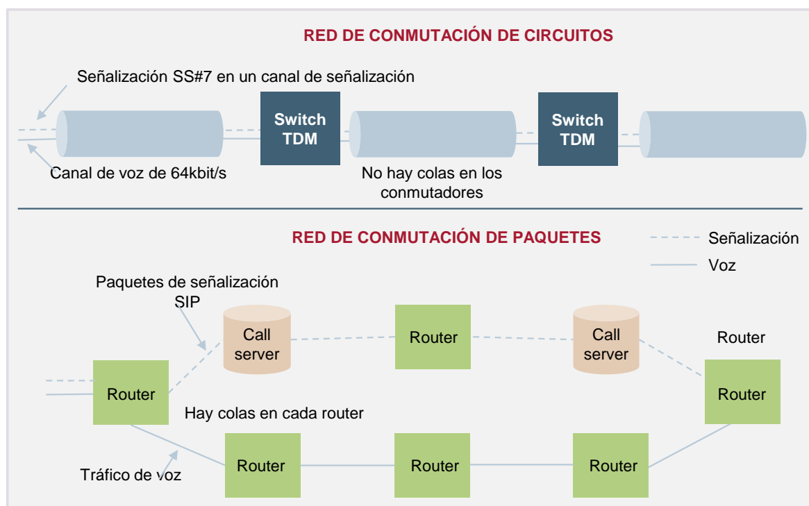
Figura 4.8: Comparación entre redes de conmutación de circuitos y de conmutación de paquetes [Fuente: Analysys Mason, 2012]
