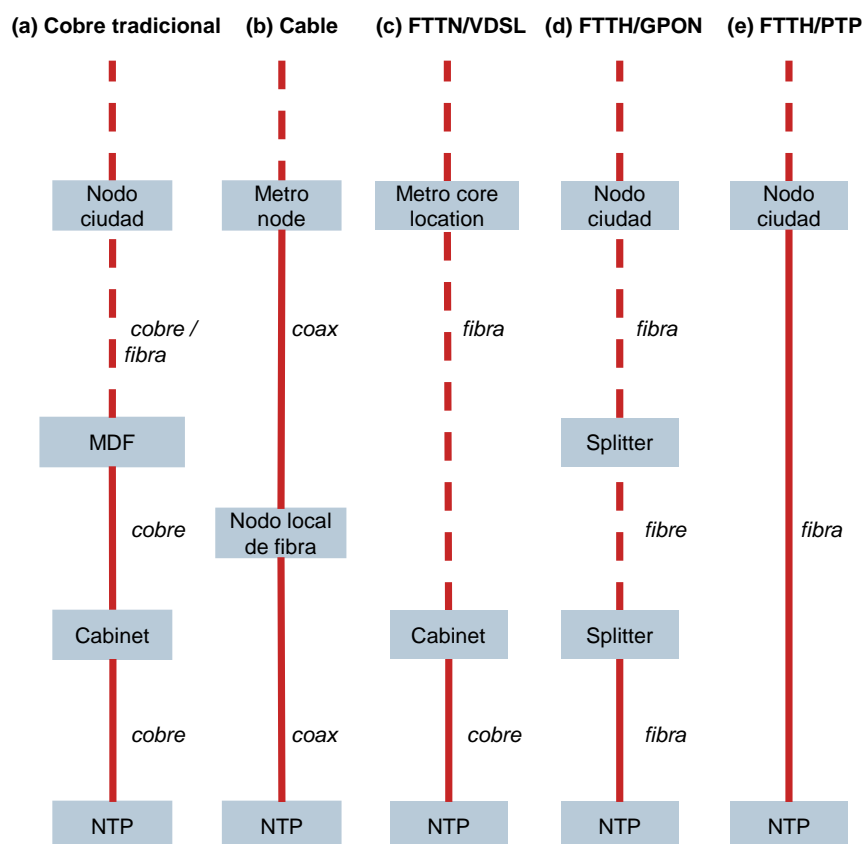
Figura 4.5: Arquitecturas de la red de acceso [Fuente: Analysys Mason, 2012]
