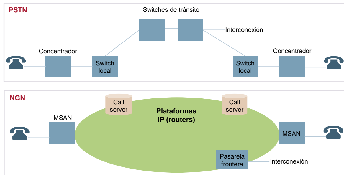
Figura 4.9: Comparación de la red PSTN tradicional y los servicios de voz sobre una NGN [Fuente: Analysys Mason, 2012]
