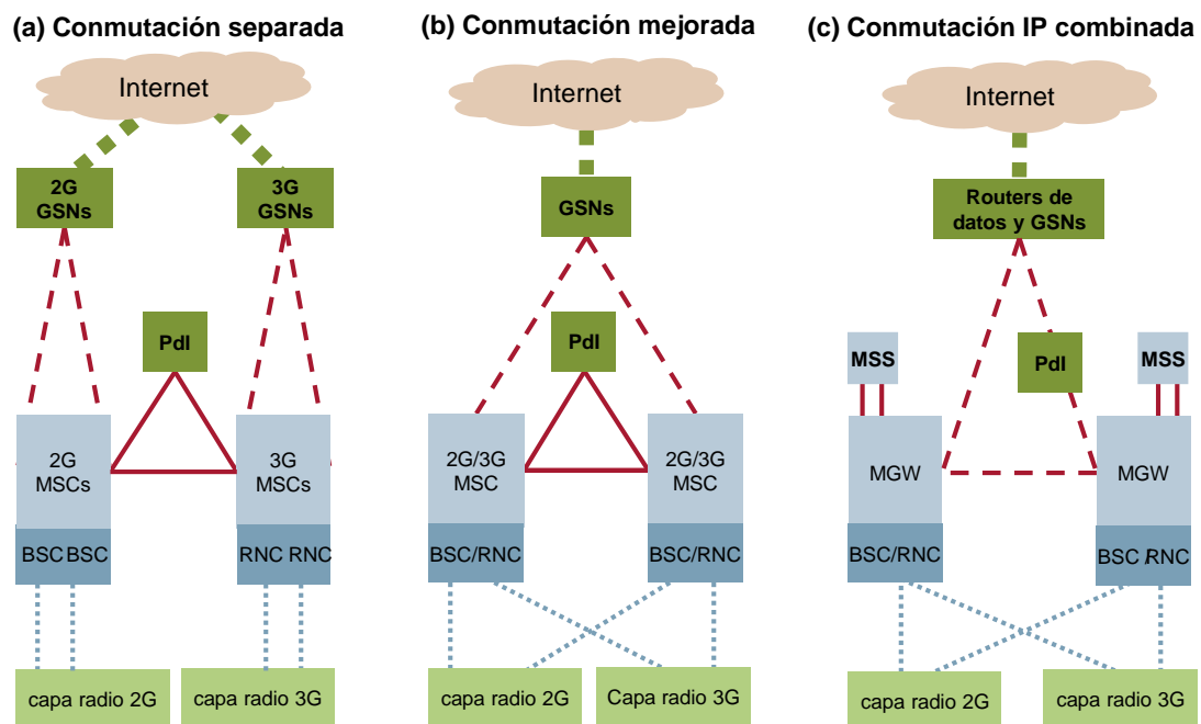
Figura 4.4: Opciones de arquitectura para el modelo BULRIC móvil [Fuente: Analysys Mason, 2012]
