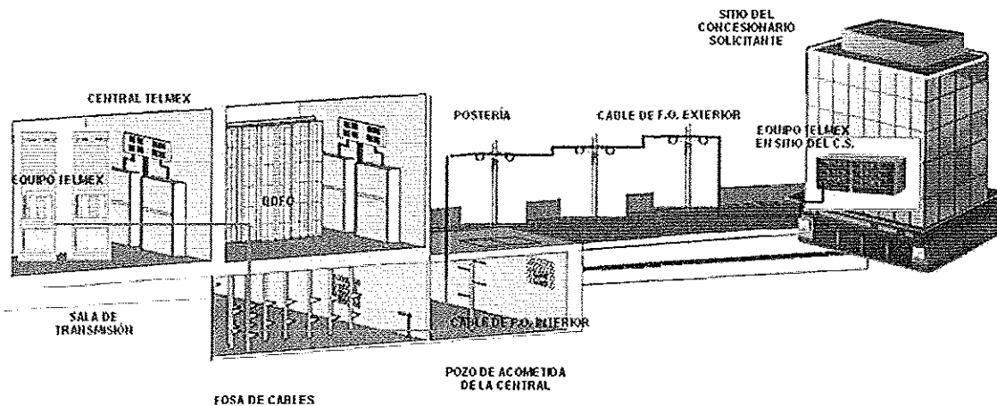
Figura 4. Lada Enlace con FO aérea
