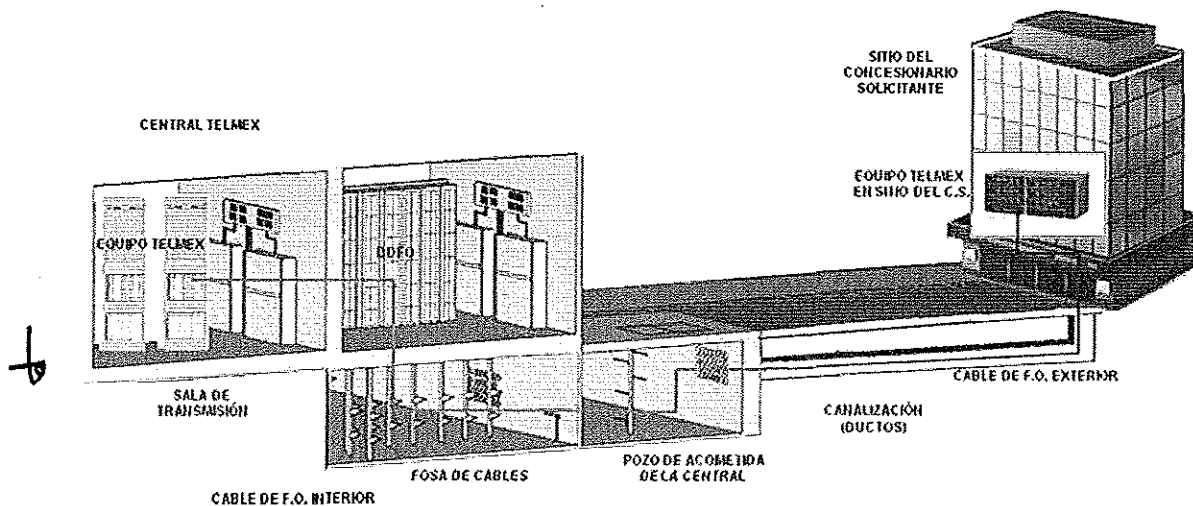
Figura 3. Lada Enlace con FO canalizada
