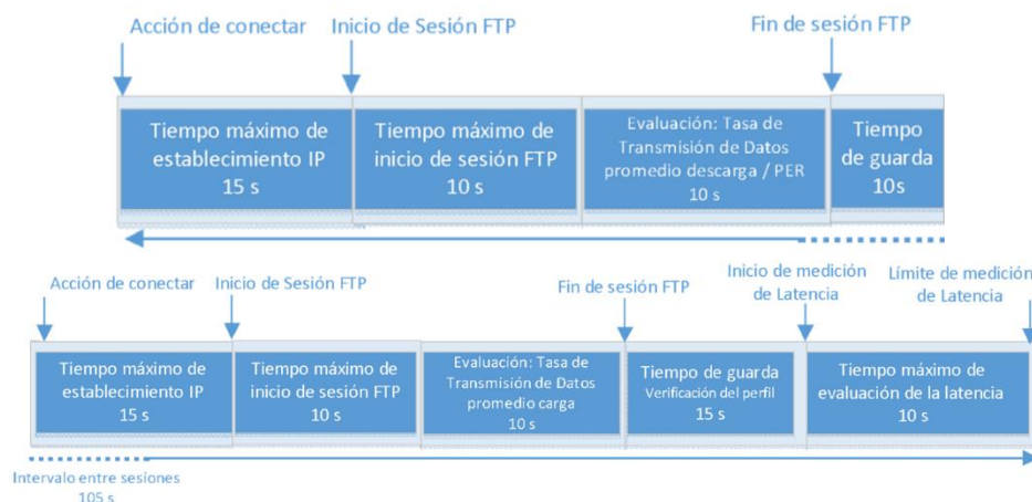
Imagen 7. Diagrama de la secuencia para evaluar los parámetros de calidad del Servicio de Transferencia de Datos
