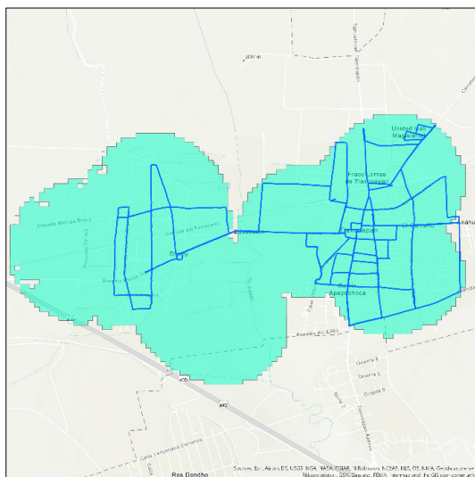
Imagen 2 a). Intersección de los mapas de cobertura garantizada, de todos los concesionarios y OMV, y recorrido de medición para los servicios de voz y SMS, en i) Tepeji del Rio de Ocampo, ii) Tula de Allende, iii) Tlaxcoapan y iv) Tizayuca.
