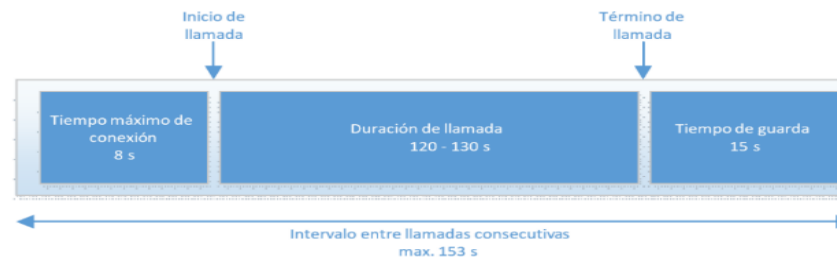
Imagen 5. Diagrama de la secuencia para evaluar los parámetros de calidad del servicio de Voz.
