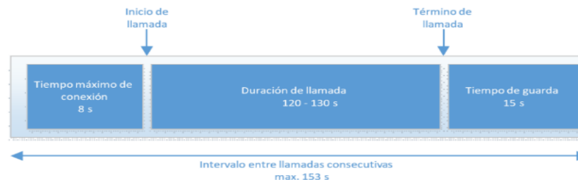
Imagen 5. Diagrama de la secuencia para evaluar los parámetros de calidad del servicio de Voz.
