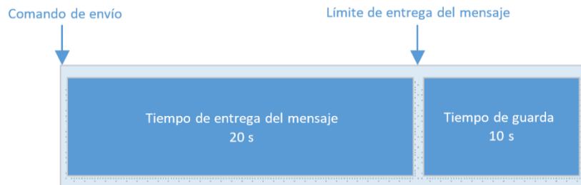
Imagen 6. Diagrama de la secuencia para evaluar los parámetros de calidad del servicio de SMS.
