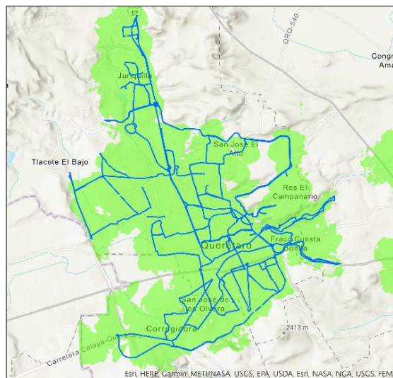
Imagen 4. Intersección de los mapas de cobertura garantizada y recorrido de medición para la tecnología de acceso LTE, de todos los concesionarios y OMV, en i) Santiago de Querétaro.
