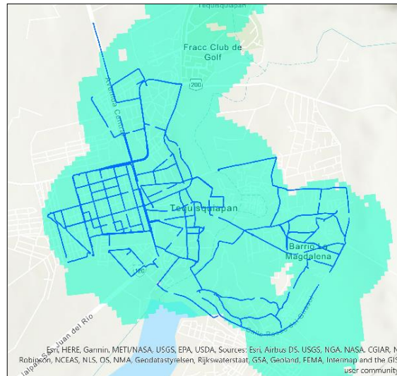
Imagen 2. Intersección de los mapas de cobertura garantizada, de todos los concesionarios y OMV, y recorrido de medición para los servicios de voz y SMS, en i) Santiago de Querétaro, ii) Pedro Escobedo, iii) San Juan del Río y iv) Tequisquiapan.
