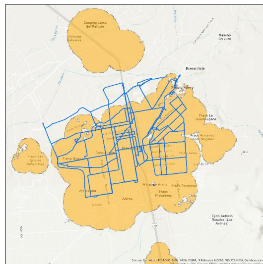
Imagen 3. Intersección de los mapas de cobertura garantizada y recorrido de medición para la tecnología de acceso 3G, de todos los concesionarios y OMV, en i) Hermosillo, ii) Cd. Obregón y iii) Navojoa.
