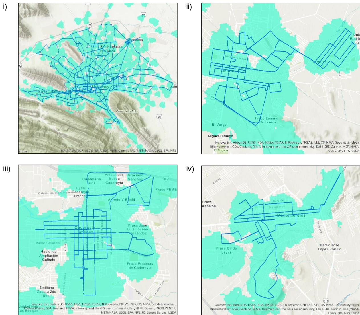
Imagen 2. Intersección de los mapas de cobertura garantizada, de todos los concesionarios y OMV, y recorrido de medición para los servicios de voz y SMS, en i) Monterrey, San Pedro Garza García, San Nicolás de los Garza, Santa Catarina, Guadalupe y Apodaca, ii) Linares, iii) Cadereyta Jiménez y iv) Montemorelos.
