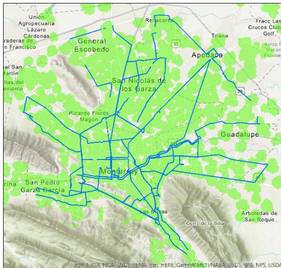
Imagen 4. Intersección de los mapas de cobertura garantizada y recorrido de medición para la tecnología de acceso LTE, de todos los concesionarios y OMV, en i) Monterrey, San Pedro Garza García, San Nicolás de los Garza, Santa Catarina, Guadalupe y Apodaca, y ii) Cadereyta Jiménez.
