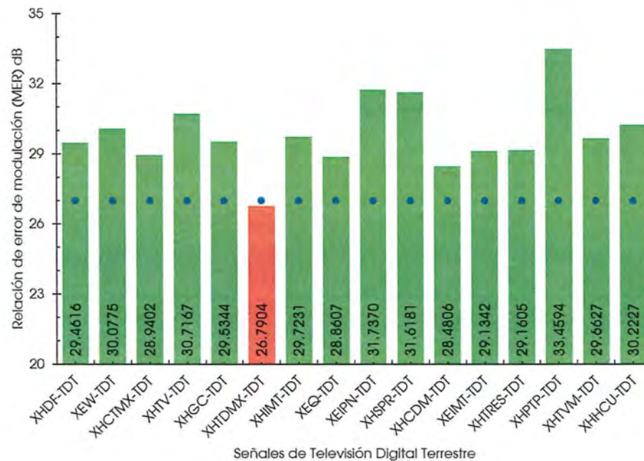
Gráfico 1. Valores promedio del parámetro de calidad MER y valor mínimo aceptable del parámetro
