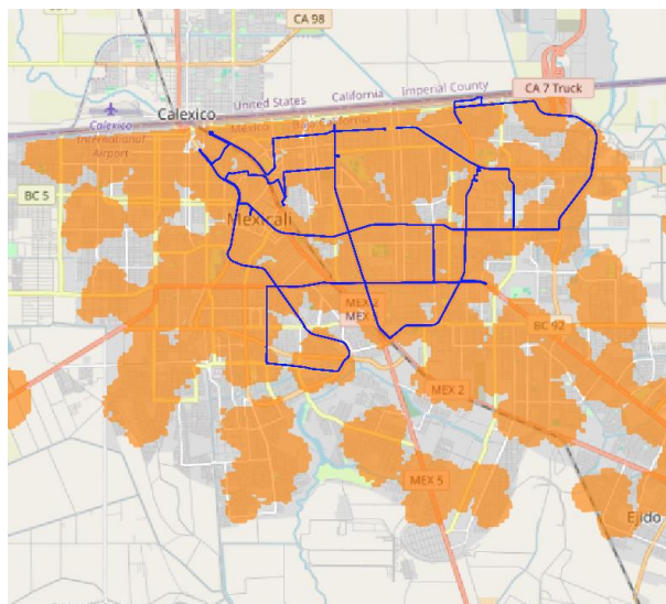
Imagen 3). Mapa resultante de la intersección de la cobertura garantizada y recorrido de medición para la tecnología de acceso 3G, de todos los Concesionarios y OMV, en i) Ensenada, ii) Tijuana y iii) Mexicali.
