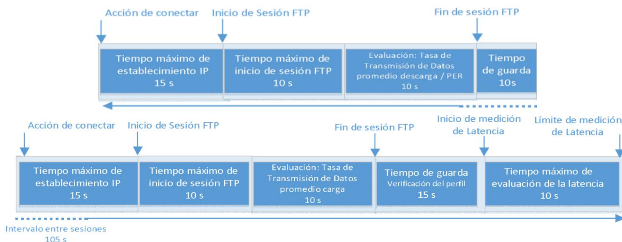
Imagen 7. Diagrama de la secuencia para evaluar los parámetros de calidad del Servicio de Transferencia de Datos
