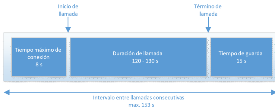
Imagen 4. Diagrama de la secuencia para evaluar los parámetros de calidad del servicio de Voz.
