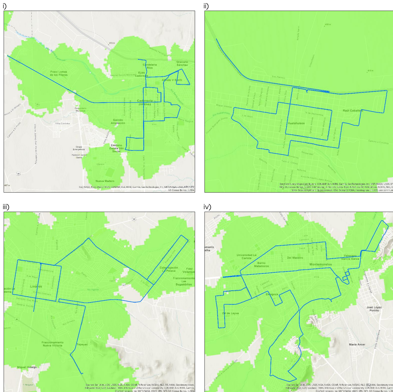
Imagen 4a). Mapa resultante de la intersección de la cobertura garantizada y recorrido de medición para la tecnología de acceso LTE, de todos los Concesionarios y OMV, en i) Cadereyta Jiménez, ii) Hualahuis, iii) Linares y, iv) Montemorelos.
