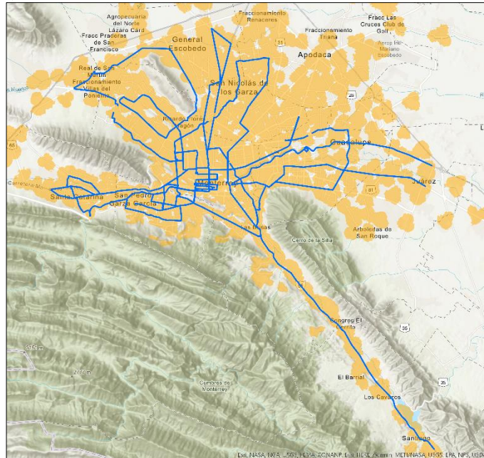
Imagen 3b). Mapa resultante de la intersección de la cobertura garantizada y recorrido de medición para la tecnología de acceso 3G, de todos los Concesionarios y OMV, en iii) Linares, iv) Montemorelos y, v) Zona metropolitana de Monterrey.
