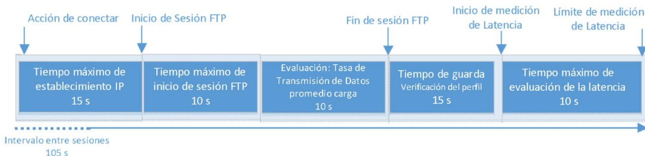
Imagen 7. Diagrama de la secuencia para evaluar los parámetros de calidad del Servicio de Transferencia de Datos
