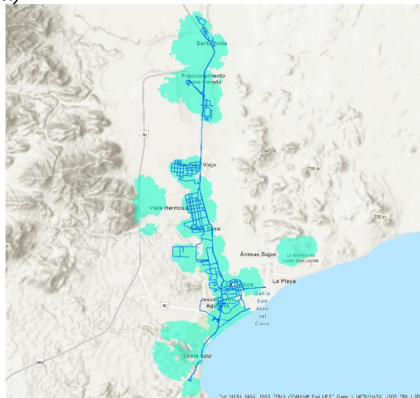
Imagen 2. Mapas de cobertura garantizada, de todos los concesionarios y OMV, y recorridos de medición para los servicios de Voz y SMS en i) El Centenario, ii) El Triunfo, iii) Los Barriles, iv) Los Cabos, v) La Paz, vi) San José del Cabo
