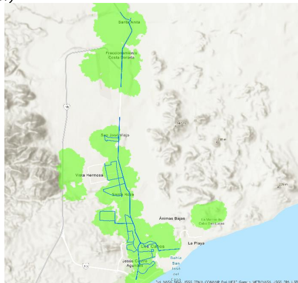
Imagen 4 Mapa de cobertura garantizada y recorrido de medición para la tecnología de acceso LTE, de todos los concesionarios y OMV, en i) El Centenario, ii) Los Cabos, iii) La Paz, iv) San José del Cabo
