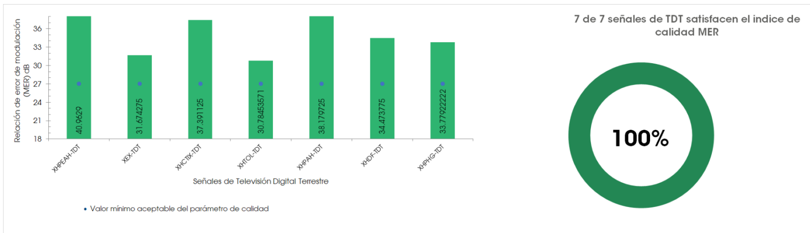
Gráfico 1. Valores promedio del parámetro de calidad MER y valor mínimo aceptable del parámetro
