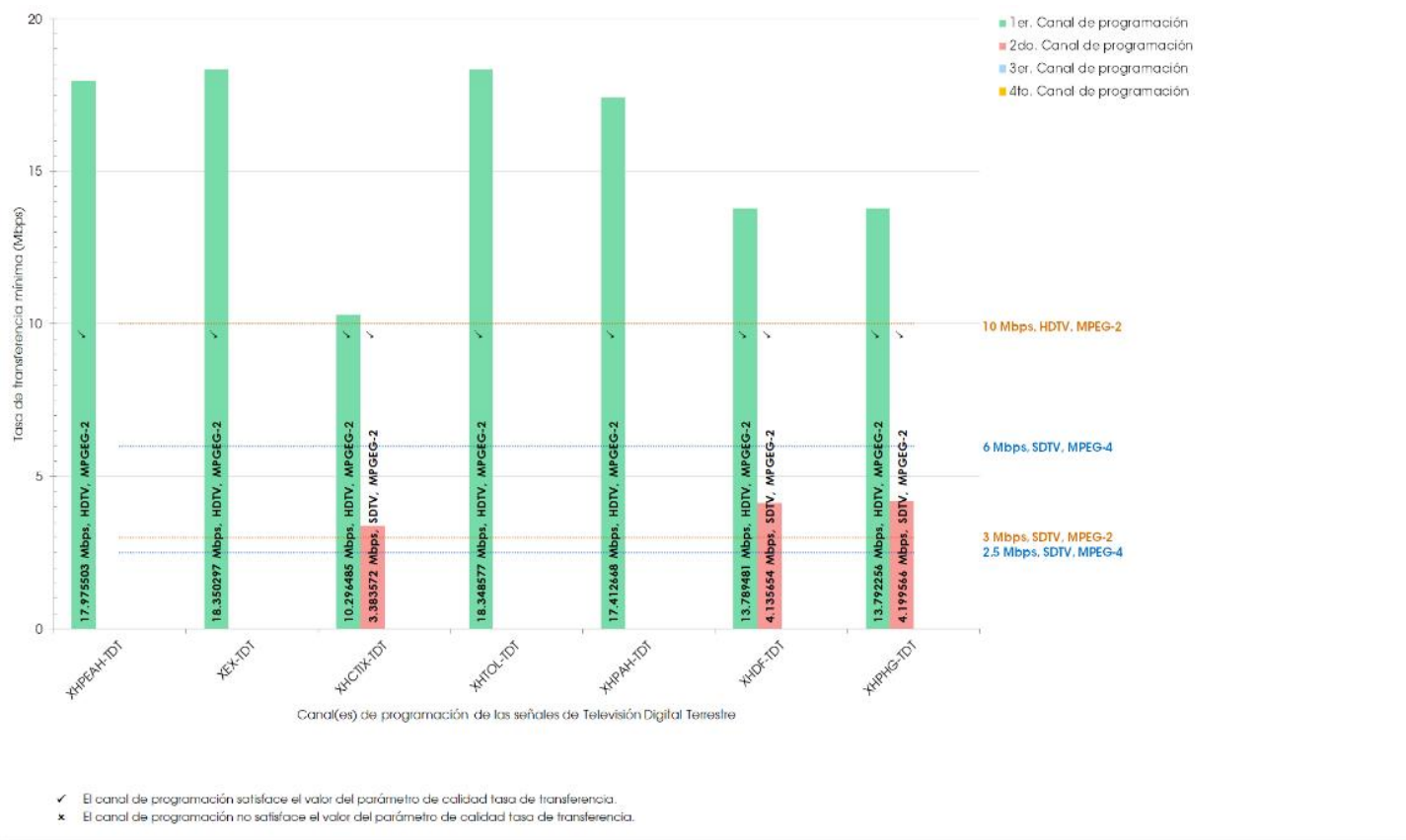
Gráfico 3. Valor del parámetro de calidad tasa de transferencia, por canal de programación de las señales de TDT 9
