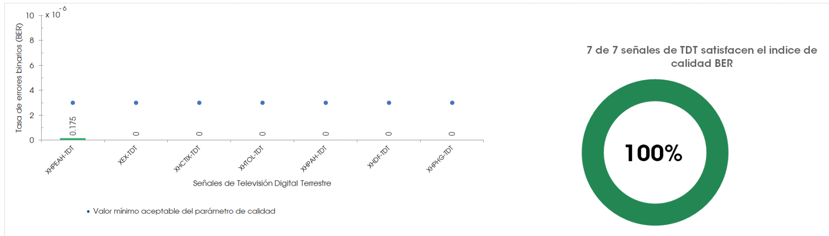
Gráfico 2. Valores promedio del parámetro de calidad BER y valor máximo aceptable del parámetro
