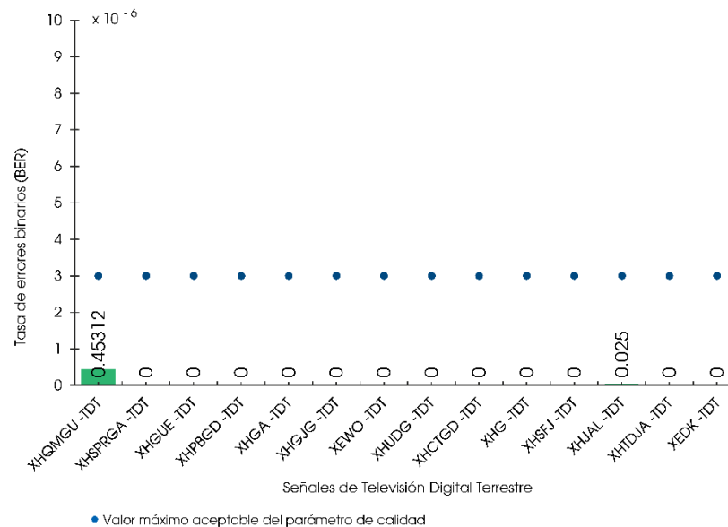
Gráfico 2. Valores promedio del parámetro de calidad BER y valor máximo aceptable del parámetro
