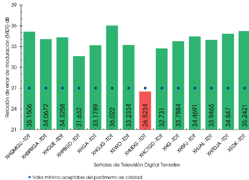
Gráfico 1. Valores promedio del parámetro de calidad MER y valor mínimo aceptable del parámetro
