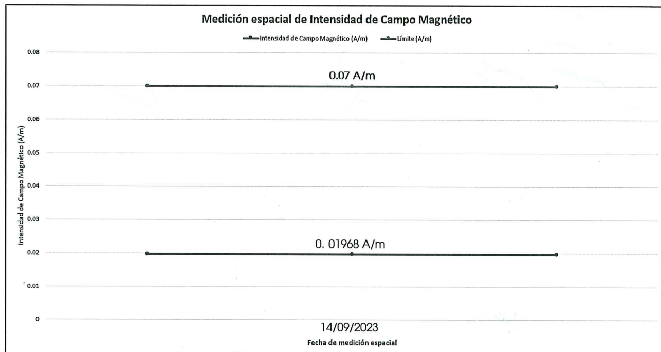
Imagen 20. Comparativo entre el valor espacial obtenido en el punto de medición 1 y el límite para campo magnético 0.073 A/m para exposición poblacional.
