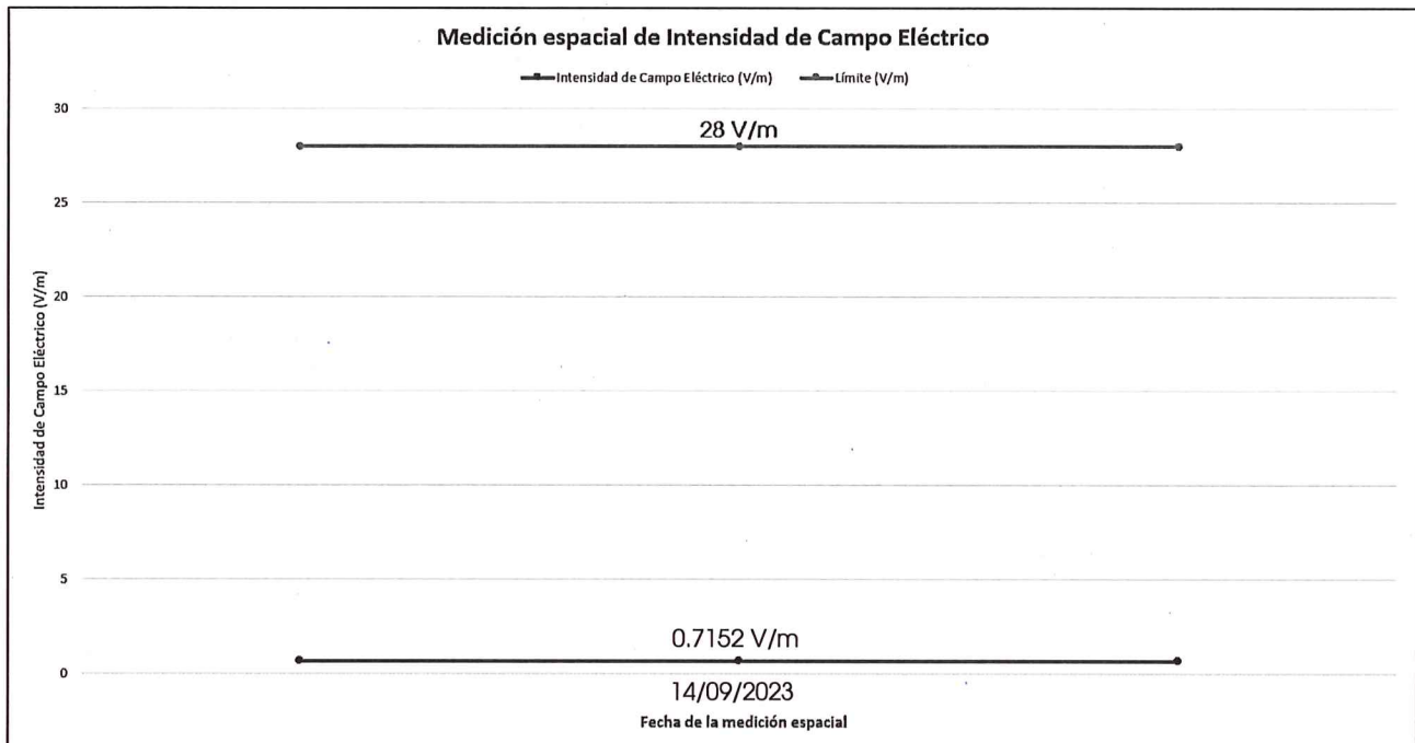
Imagen 19. Comparativo entre el valor espacial obtenido en el punto de medición 1 y el límite para campo eléctrico 28 V/m para exposición poblacional.
