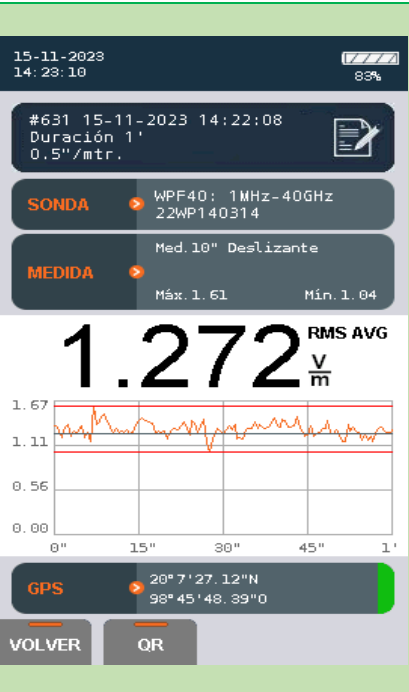
Imagen 18.-Valores de RNI obtenidos en el punto de medición 14.
