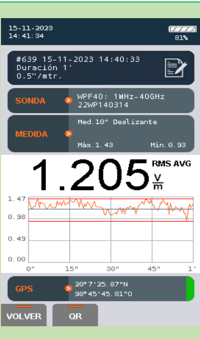
Imagen 22.-Valores de RNI obtenidos en el punto de medición 18.
