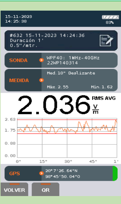
Imagen 19.-Valores de RNI obtenidos en el punto de medición 15.
