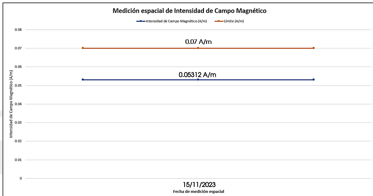
Imagen 27. Comparativo entre el valor espacial obtenido en el punto de medición 7 y el límite para campo magnético 0.073 A/m para exposición poblacional.
