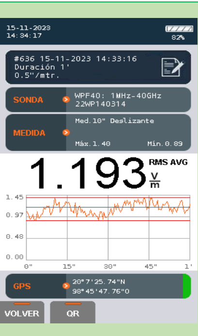
Imagen 21.-Valores de RNI obtenidos en el punto de medición 17.
