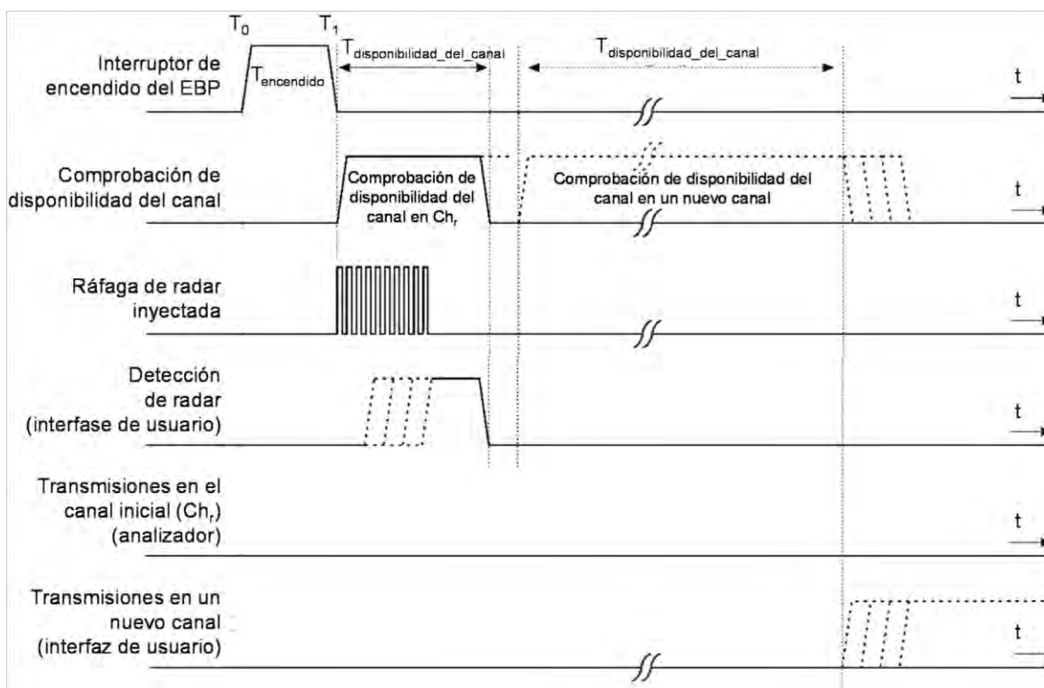
Figura 27. Ejemplo de diagrama de tiempo para las pruebas de radar al comienzo del tiempo de comprobación de disponibilidad del Canal.
