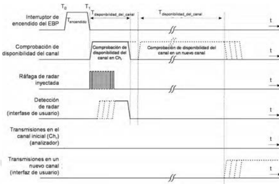
Figura 9. Ejemplo de la traza de tiempo para las pruebas de radar al comienzo del tiempo de comprobación de disponibilidad del Canal.
