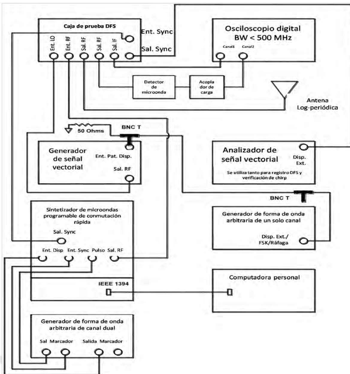
Figura 21a. Ejemplo de generador de forma de onda de radar de Pulso corto y largo.
