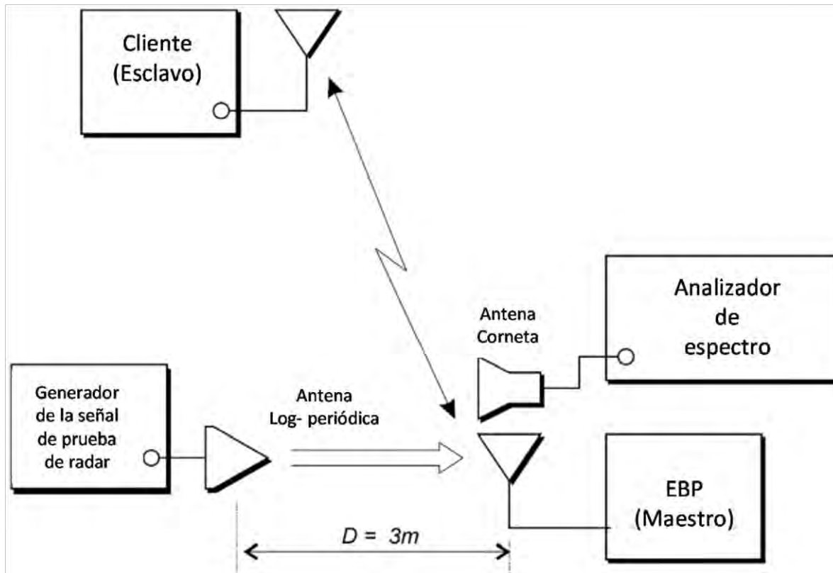
Figura 17. Ejemplo de configuración radiada donde el EBP es un Maestro y las formas de onda de prueba de radar se inyectan en el Maestro.
