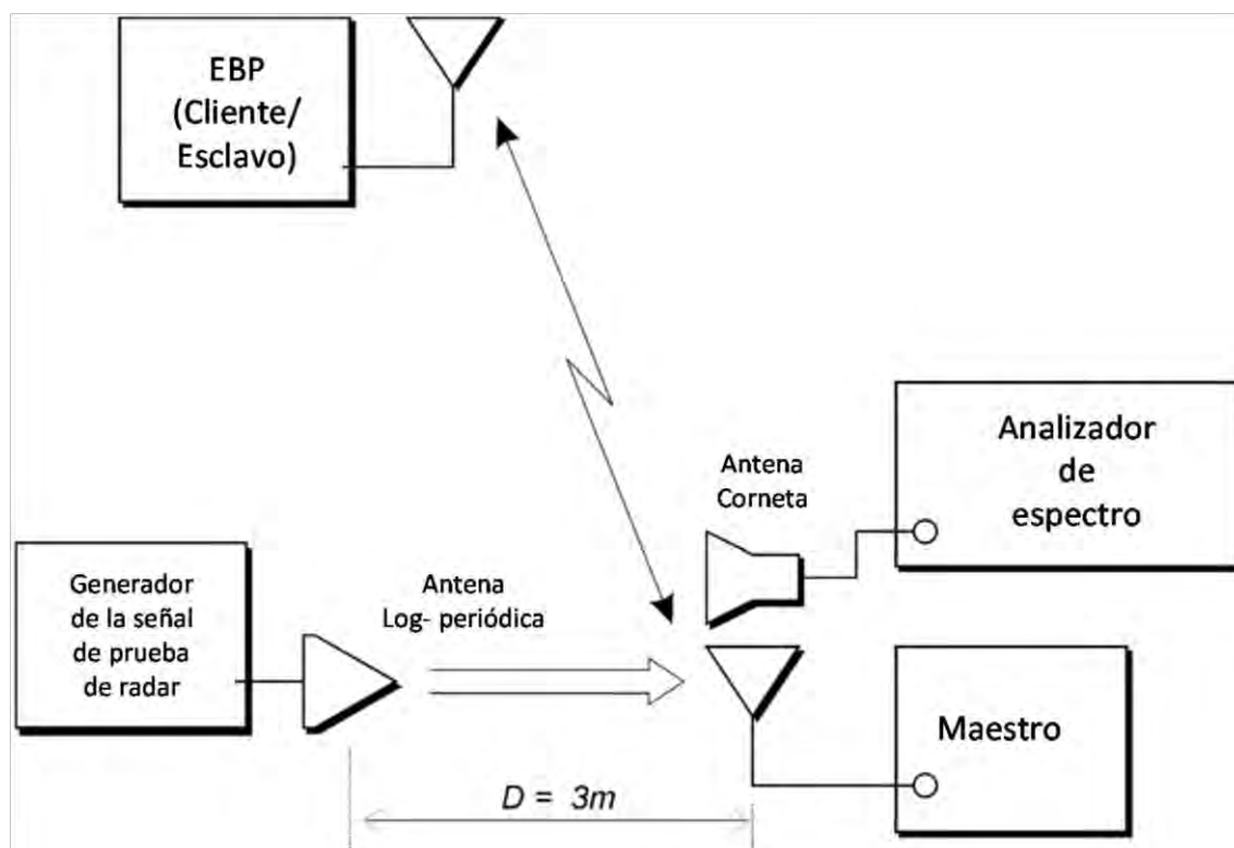
Figura 18. Ejemplo de configuración radiada donde el EBP es un Cliente y se inyectan formas de onda de prueba de radar en el Maestro.
