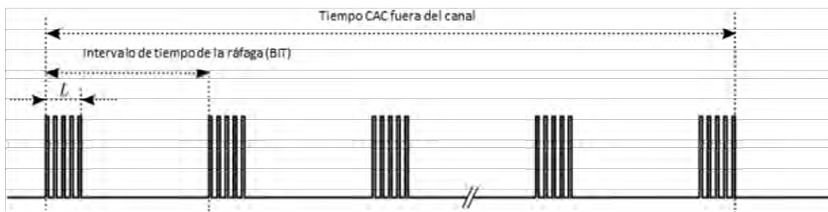
Figura 2B. Estructura general de la señal de prueba de radar de múltiples ráfagas/ basada en PRF constante.
