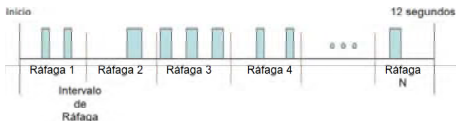
Figura 3. Representación gráfica de una forma de onda de tipo radar de Pulso largo
