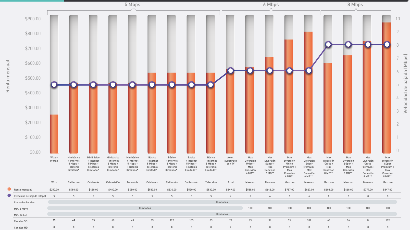
Gráfico 12. Renta mensual y principales variables en planes con velocidad de bajada de 4 Mbps y menor a 10 Mbps
