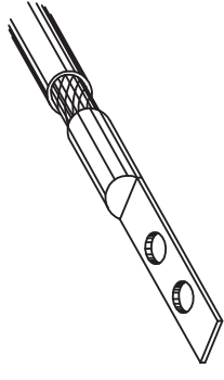
ZAPATA PONCHABLE DE 2 OJILLOS
