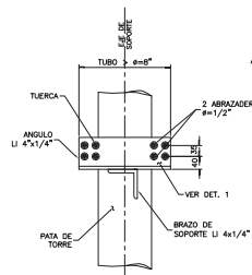
- CORTE B-B -
