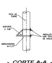
- CORTE A-A -
