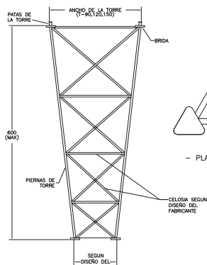
- BASE CONICA -
