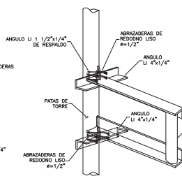
- ISOMETRICO -
