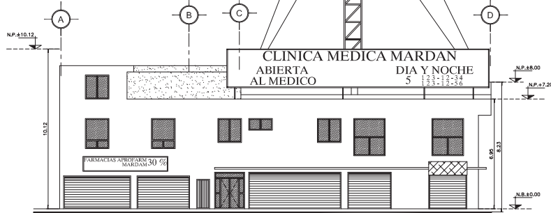
FACHADA ESTE
