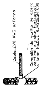
SOLDADURA CADWELD TIPO RJ
