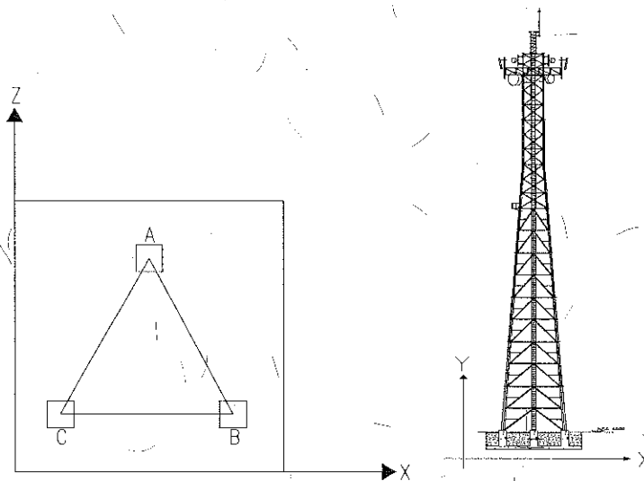
ORIENTACION DEL MODELO DE LA ESTRUCTURA EN EL SOFTWARE STAAD.PRO
