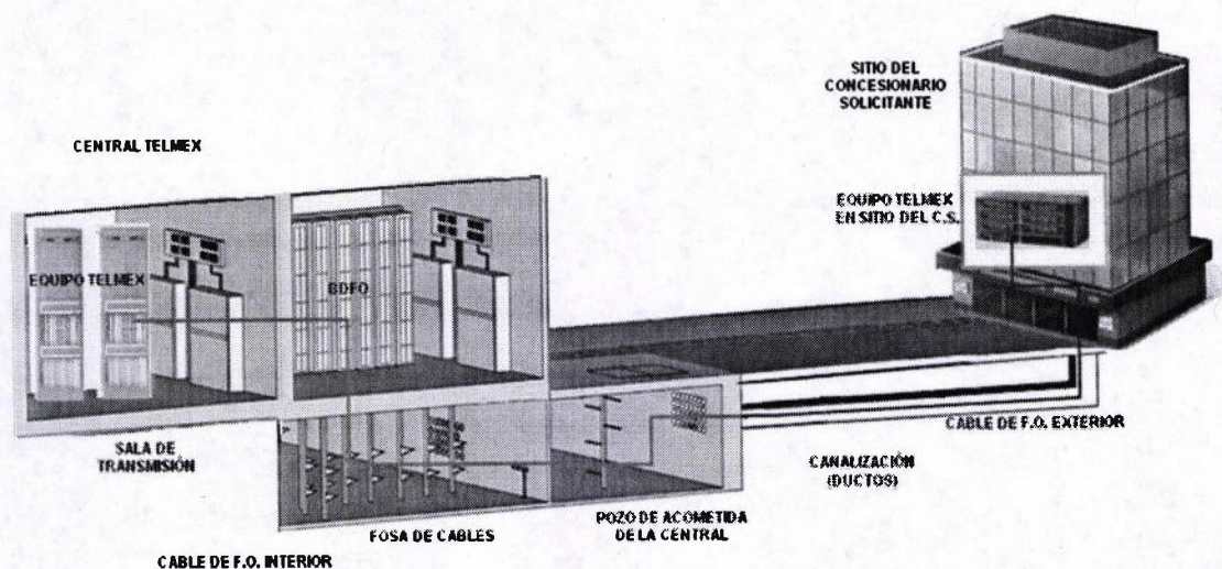
Figura 3. Lada Enlace con FO canalizada
