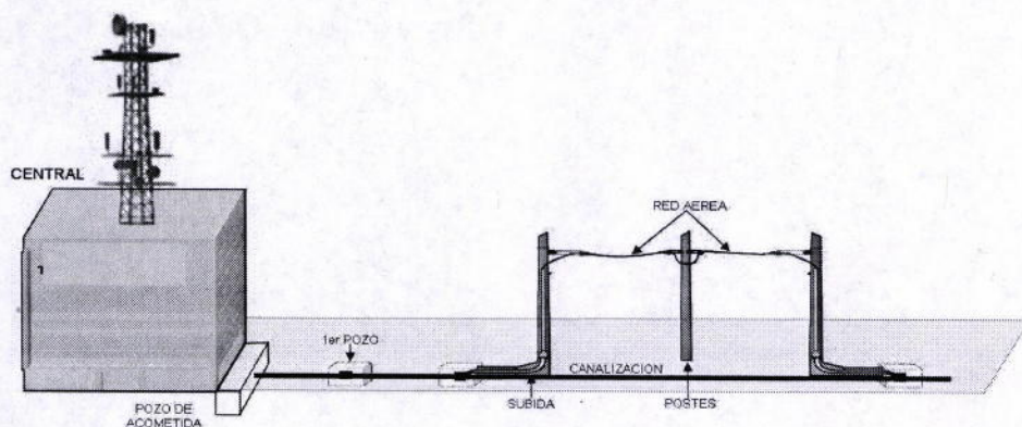
Figura 1 Edificio, Torre, y Obra Civil de Telnor.
