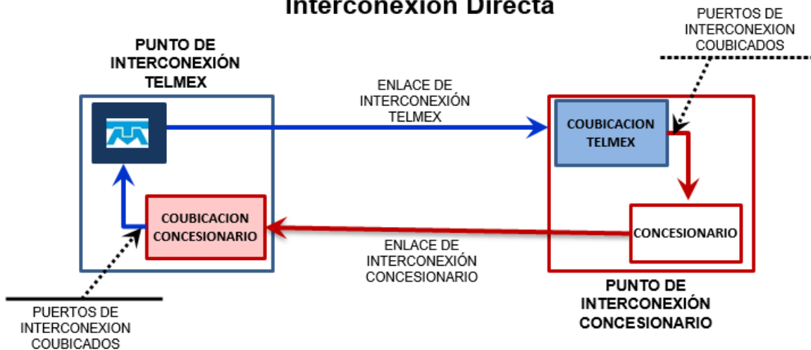
Diagrama de Interconexión para señalización SIP
