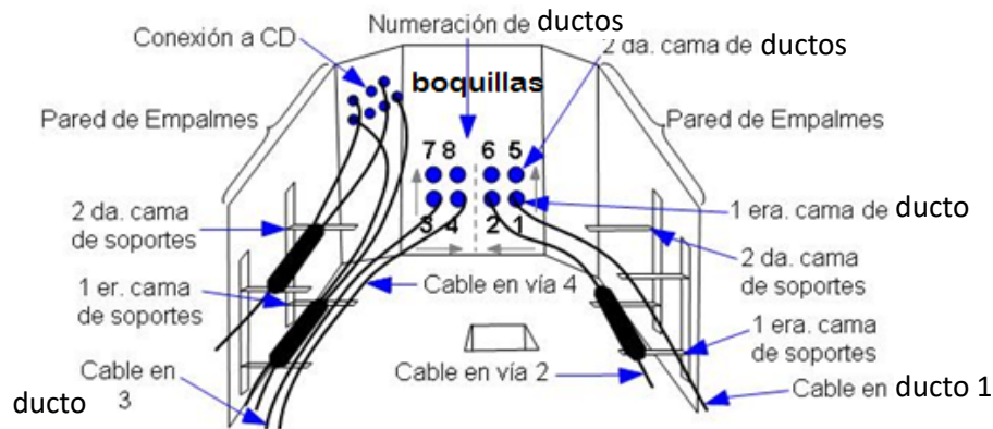
Figura 2. Ocupación de ductos y soportes de cables en pozos con dos paredes de empalme.
