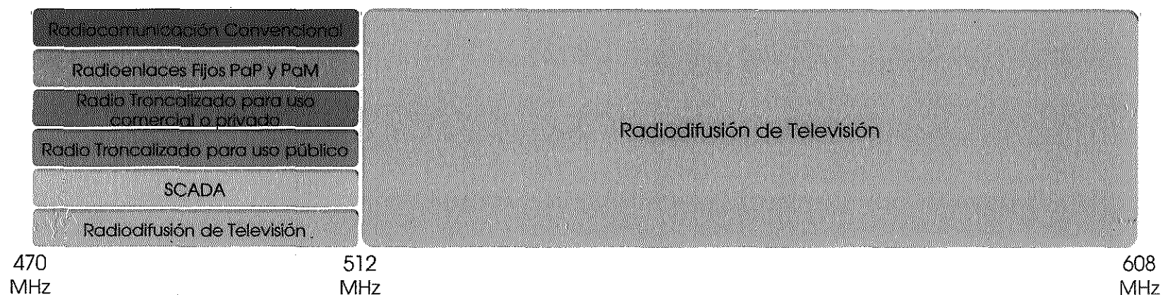
Figura 5. Distribución actual de la banda 470 – 608 MHz
