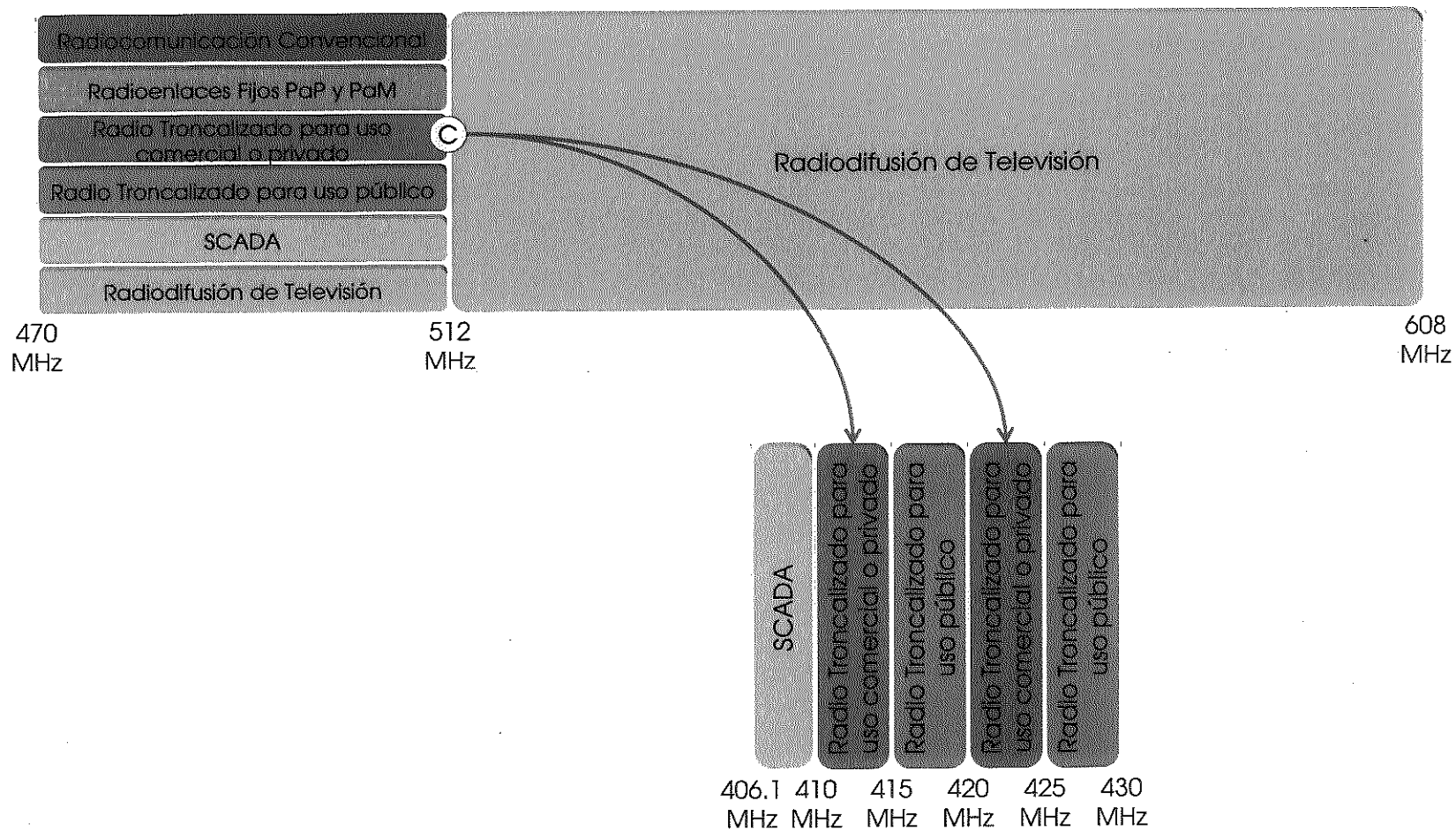
Figura 9. Ejemplificación de despeje y migración para aplicaciones de radio troncalizado para uso comercial o privado.
