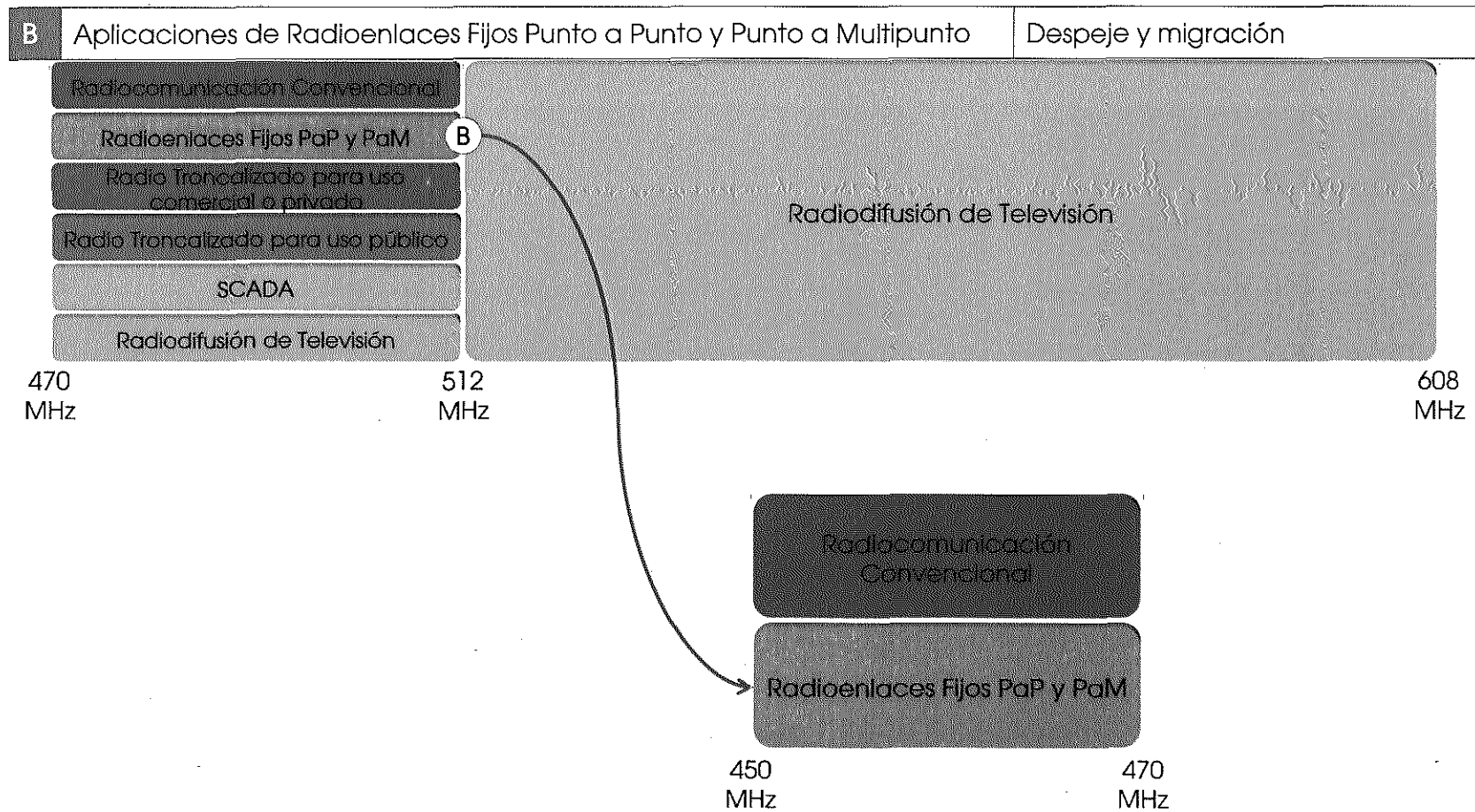
Figura 8. Ejemplificación de despeje y migración para aplicaciones de radioenlaces fijos punto a punto y punto a multipunto.
