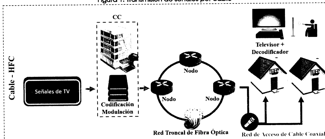
Figura 1. Transmisión de señales por cable
