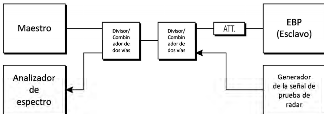
Figura 7. Configuración B.
