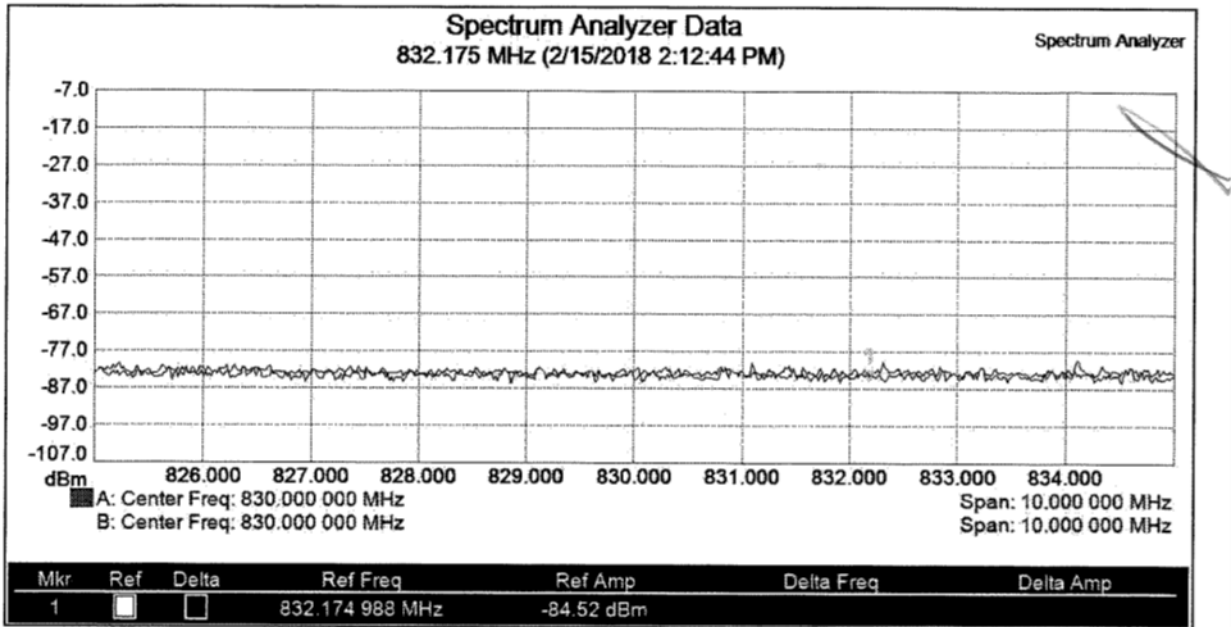
Gráfica 1. La cual abarca el rango de operación de 825 a 835 MHz y no se observa señal interferente debido al apagado del equipo repetidor que generaba la señal de la frecuencia central 832.175 MHz.
