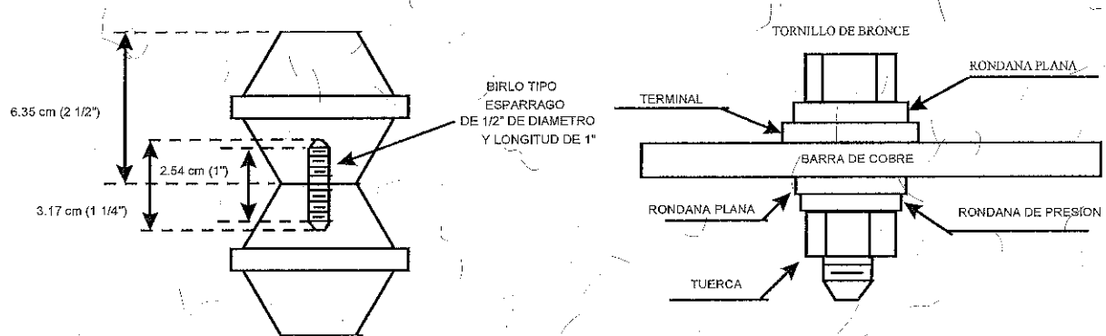
Tornillería en Barra de Cobre y entre Aisladores
