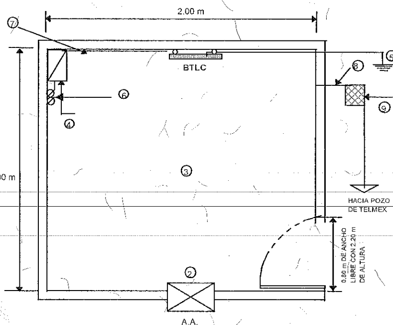
Sala con Equipo de Transmisión y Fuerza Para Fibra Óptica R.D.A.
