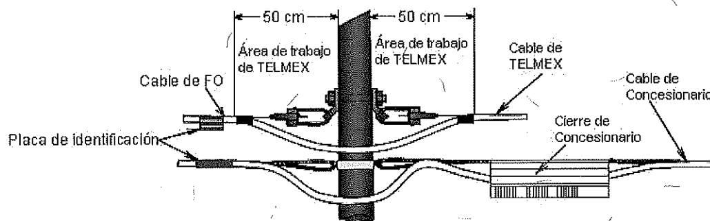
Figura 3. Cables de Telmex y Concesionario o Autorizados solicitante en postes de Telmex.
