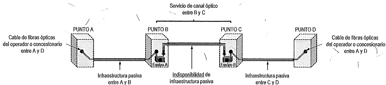
Figura 2 Compartición de infraestructura pasiva con servicio de canal óptico complementario.
