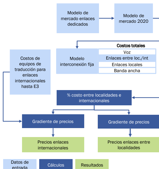
Figura 2. Esquema del modelo de enlaces dedicados
