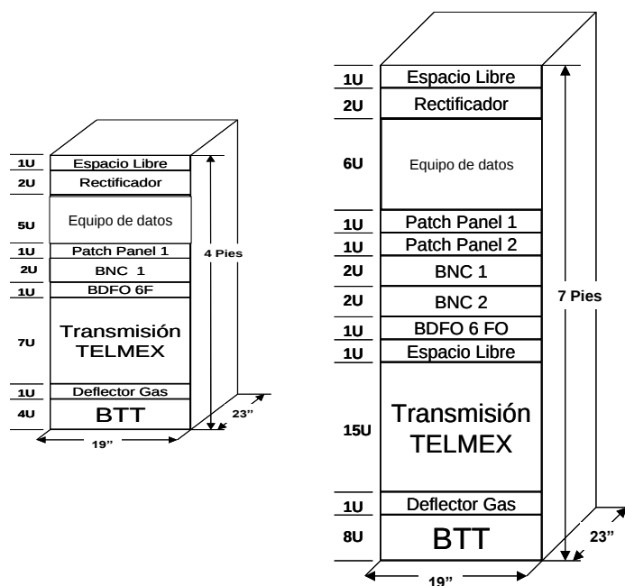
Distribución del gabinete universal Telmex/Telnor
