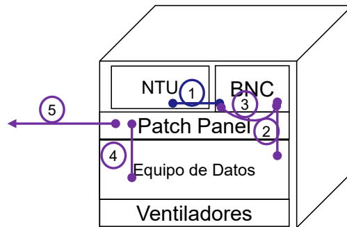
Responsabilidad de cableados en GUT y MIDI-GUT
