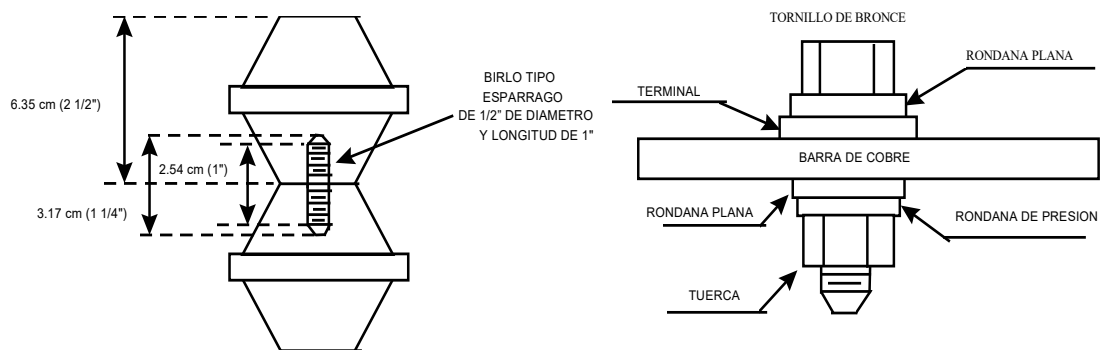
Tornillería en Barra de Cobre y entre Aisladores
