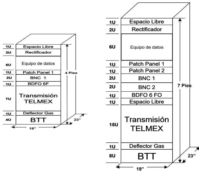
Distribución del gabinete universal Telmex
