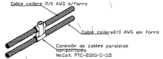
SOLDADURA CADWELD TIPO PT
