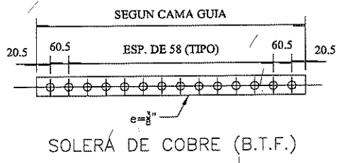
DETALLE DE KIT DE ATERRIZAJE DE FEEDERS EN CAMA GUIA DE ONDA CON BARRAS DE COBRE
