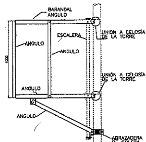
VISTA A'-A'
