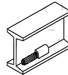
SOLDADURA CADWELD TIPO ST
