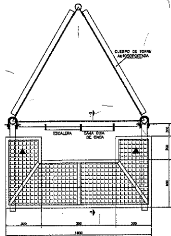
PLATAFORMA DE DESCANSO
