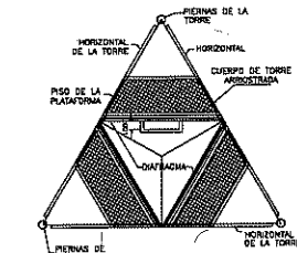
PLATAFORMA DE DESCANSO INTERIOR A LA TORRE
