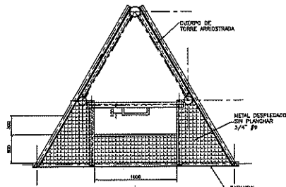
PLATAFORMA DE DESCANSO
