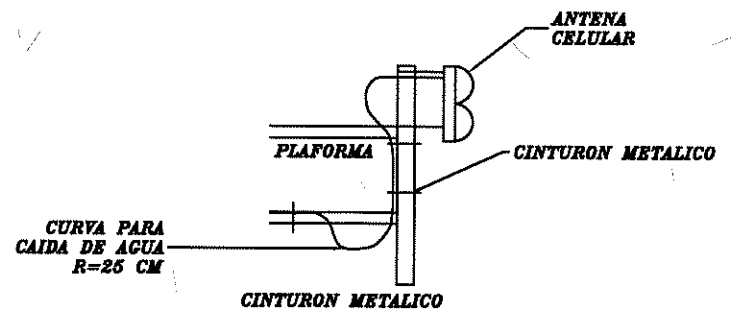
FIJACION DE FEEDERS Y JUMPER EN PLATAFORMA
