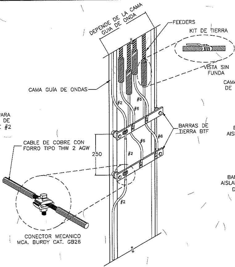
DETALLE DE KIT DE ATERRIZAJE DE FEEDERS EN CAMA GUIA DE ONDA CON BARRAS DE COBRE
