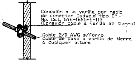
SOLDADURA CADWELD TIPO GY
