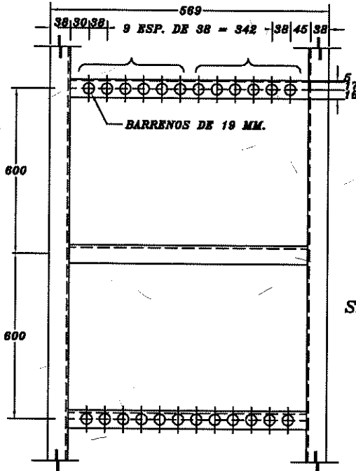
CAMA GUIA DE 12 BARRENOS (PLANTA)
