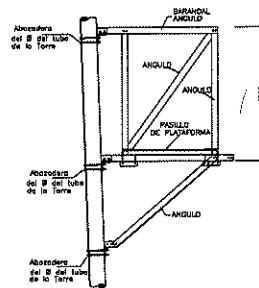
VISTA B-B'
