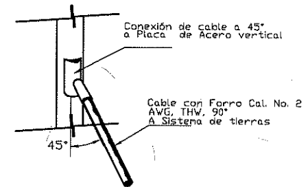
SOLDADURA CADWELD TIPO VS
