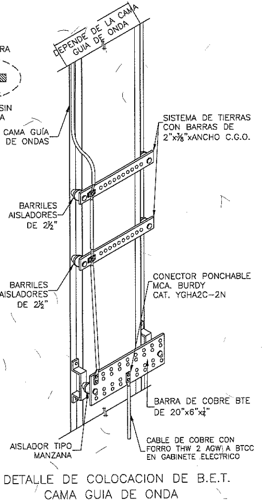
DETALLE DE KIT DE ATERRIZAJE DE FEEDERS EN CAMA GUIA DE ONDA CON BARRAS DE COBRE
