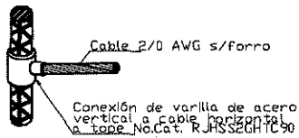
SOLDADURA CADWELD TIPO RJ
