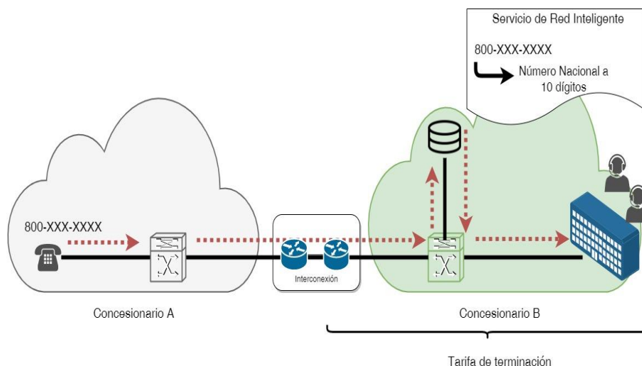
Diagrama 1. Las llamadas originadas en la red del Concesionario A con destino a un número 800 del Concesionario B son llamadas locales.
