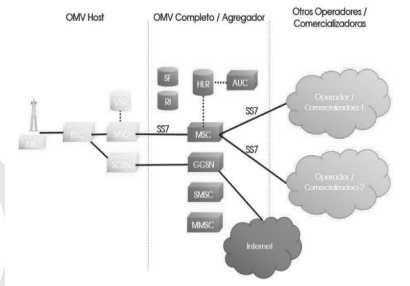
Diagrama 2. Elementos de la infraestructura de la red de un OMV Completo/Agregador
