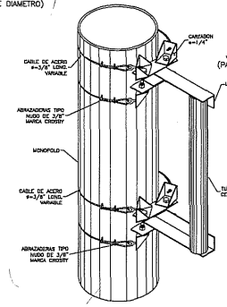
ISOMETRICO SOPORTE No. 9
