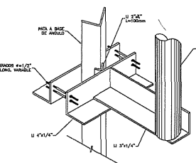
ISOMETRICO SOPORTE No. 11
