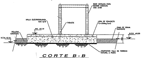
CORTE B-B
