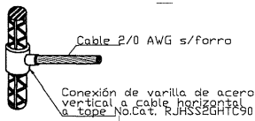
SOLDADURA CADWELD TIPO RJ
