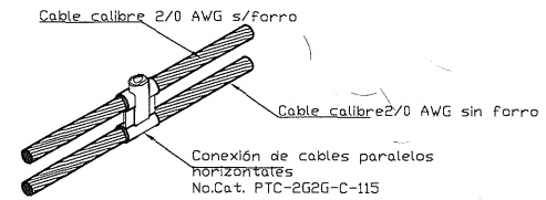
SOLDADURA CADWELD TIPO PT
