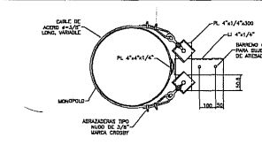
SOPORTE PARA MONOPOLO No. 10 (SOPORTE INTERMEDIO PARA SUJECION DE ATESADOR DE ANTENA, IDEM A LOS BRAZOS DEL SOPORTE No. 11, PARA INSTALACION DE ANTENAS DE 1.20m EXCLUSIVAMENTE VER NOTA No. 12)
