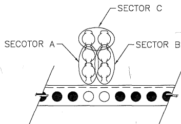
2 BARRENOS LIBRES PARA FEEDERS \phi=7/8" Y 1\ 1/4"
