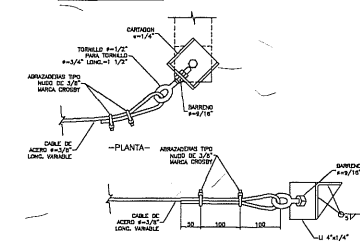
DETALLE 1
