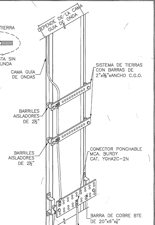
DETALLE DE COLOCACION DE B.E.T. CAMA GUIA DE ONDA
