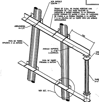
SOPORTE PARA MICROONDAS No. 12 (SOPORTE PARA TORRES AUTOSOPORTADAS Y ARRISTRADAS CON PATAS DE TUBO 4" x 2" A 10" PARA LA INSTALACION DE ANTENAS DE 1.20m A 1.80m DE DIAMETRO) NOTA: PARABRAS MAYORES A 1.00m SEAN NECESARIO EVALUAR LA COLOCACION DEL BRAZO DE CONTRAVIENTO (PUNTAJAL TUBULAR) A CELOSA DE TORRE
