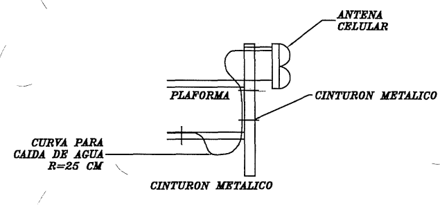
FIJACION DE FEEDERS Y JUMPER EN PLATAFORMA
