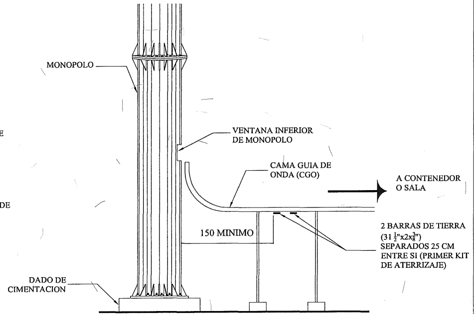
VISTA LATERAL
