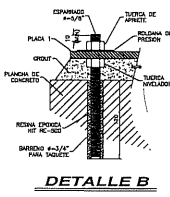
DETALLE B
