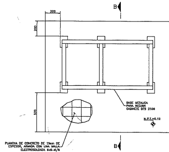
PLANCHA PARA GABINETES (PARA INSULACION EN TENDIDOS MUY ALTA Y BAJA DE GRASA)
