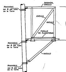
VISTA B-B'
