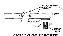
ANGULO DE SOPORTE
