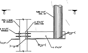
SOPORTE PARA MICROONDAS No. 11 (PARA INSTALACION DE MICROONDAS DE 0.30 A 1.20m EN TORRES TELMEJ CON PATAS A BASE DE ANGULO Y DOBLE ANGULO)
