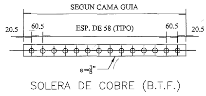
DETALLE DE KIT DE ATERRIZAJE DE FEEDERS EN CAMA GUIA DE ONDA CON BARRAS DE COBRE
