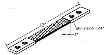
CONECTOR DE COBRE TRENZADO FLEXIBLE TIPO BD
