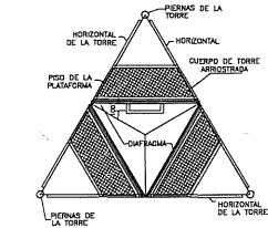
PLATAFORMA DE DESCANSO INTERIOR A LA TORRE
