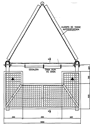
PLATAFORMA DE DESCANSO
