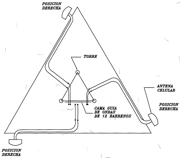
CRITERIOS DE DISTRIBUCION DE FEEDERS EN PLATAFORMAS
