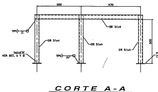
CORTE A-A
