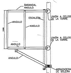
VISTA A'-A'
