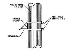
DETALLE 4
