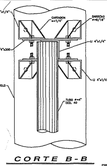
CORTE B-B
