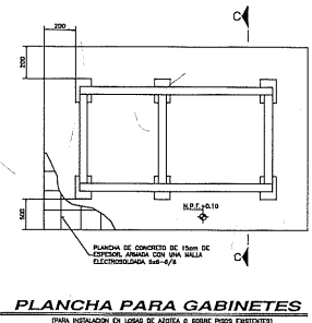
PLANCHA PARA GABINETES (PARA INSULACION EN LOSAS DE AZOTE O SOBRE PISO EXISTENTE)
