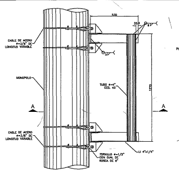
SOPORTE PARA MICROONDAS No. 9 (PARA MONOPOLOS, INSTALACION DE ANTENAS DE 0.30 A 1.20m DE DIAMETRO)
